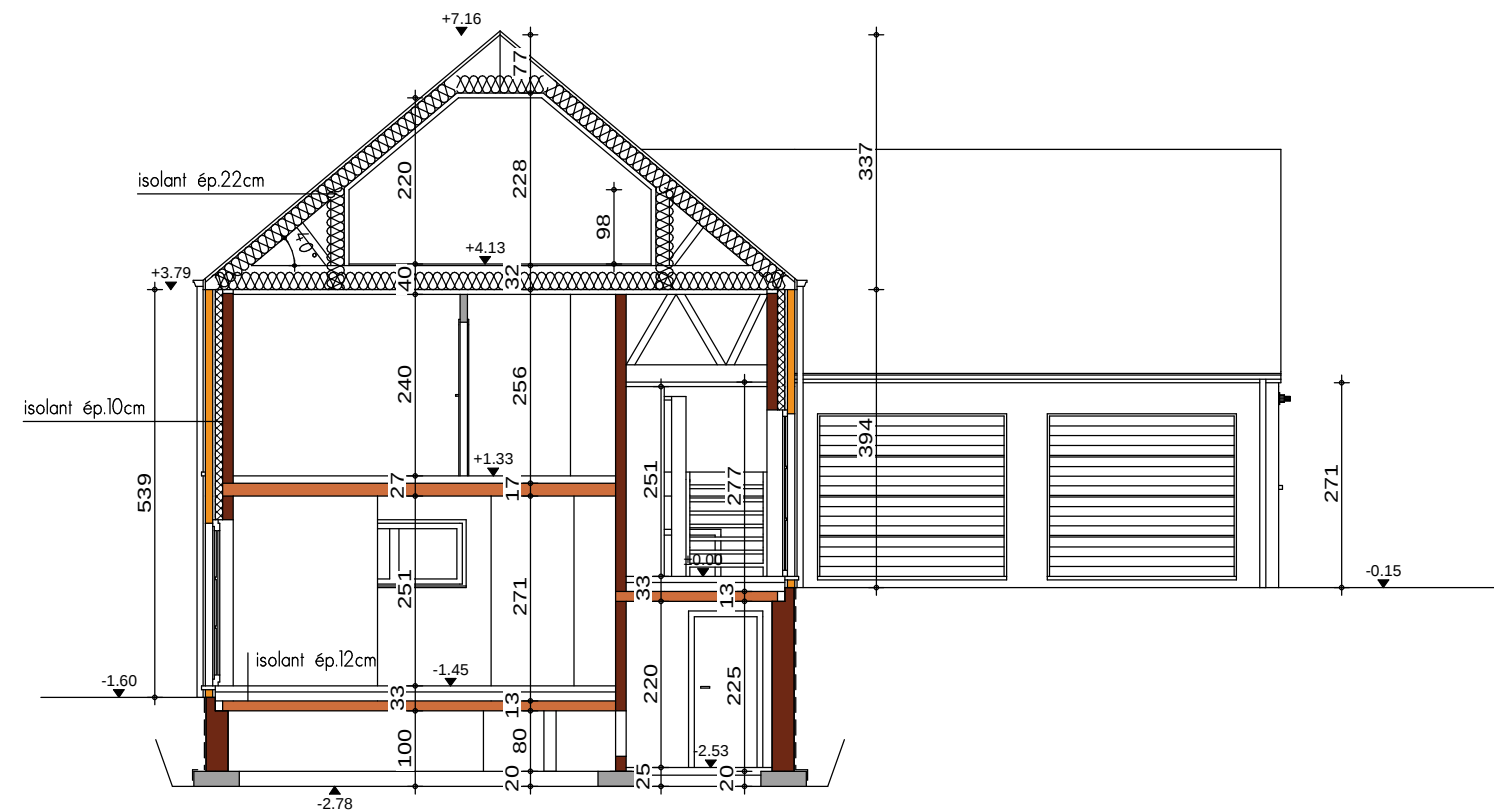
COUPE AA
