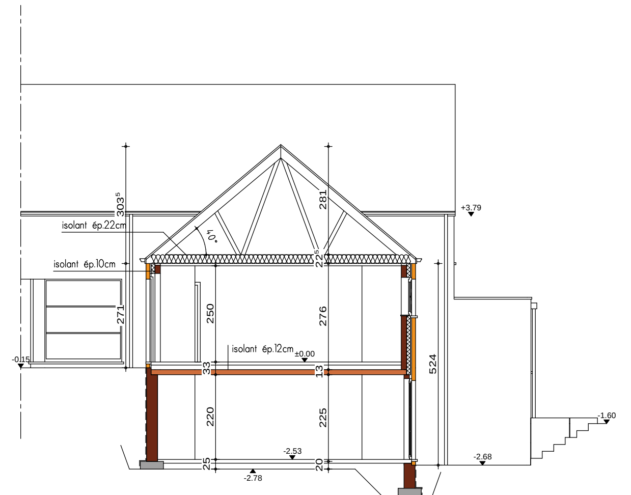
COUPE BB
