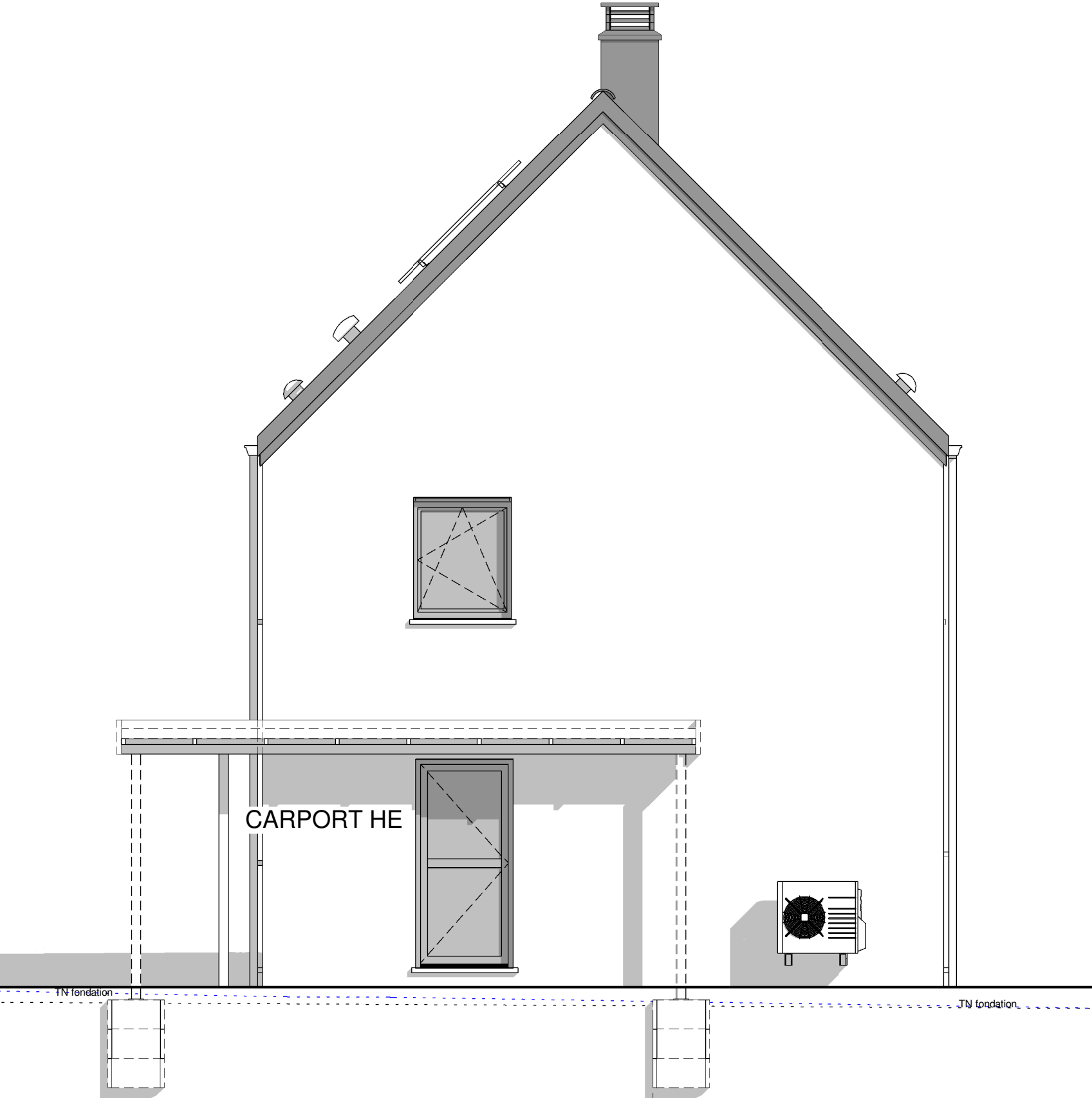
PIGNON DROIT
