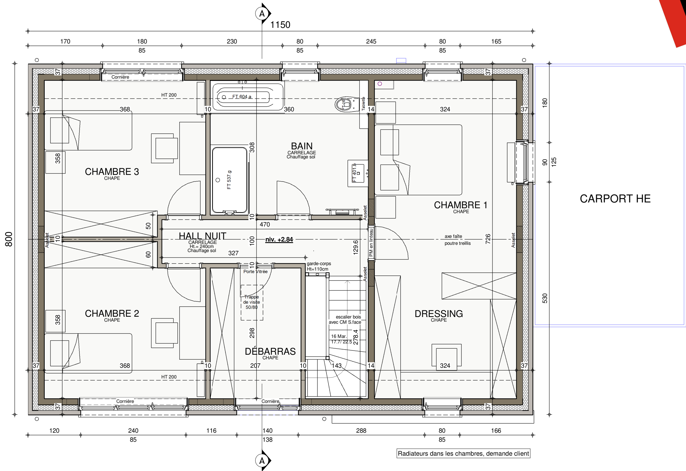
ETAGE
