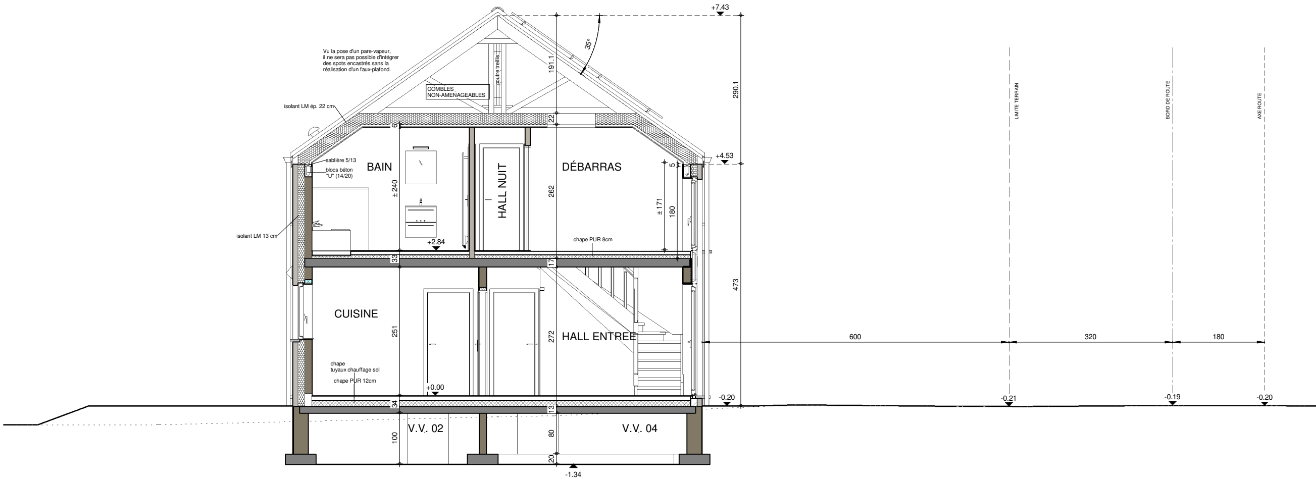
COUPE AA
