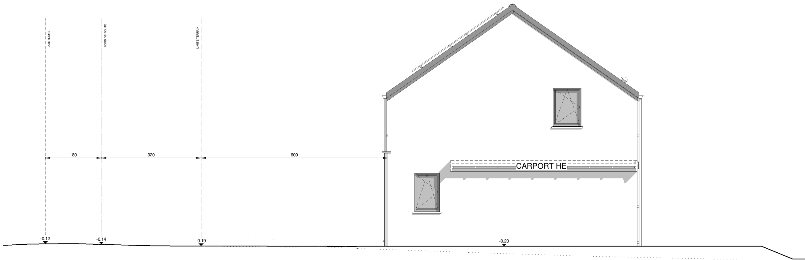
PIGNON GAUCHE
