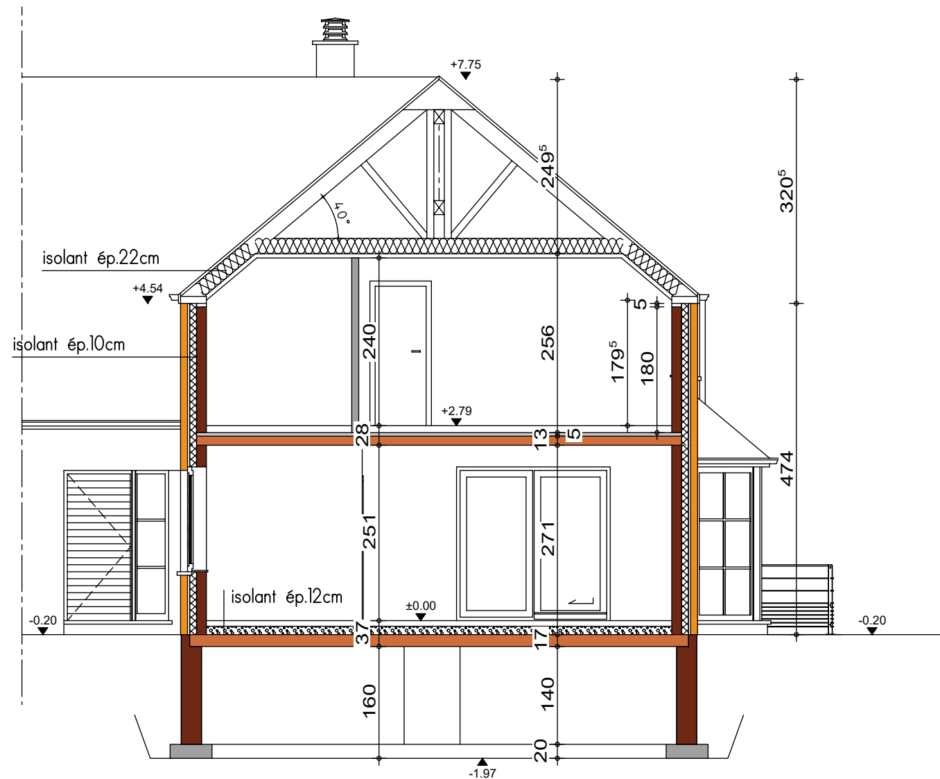
COUPE AA
