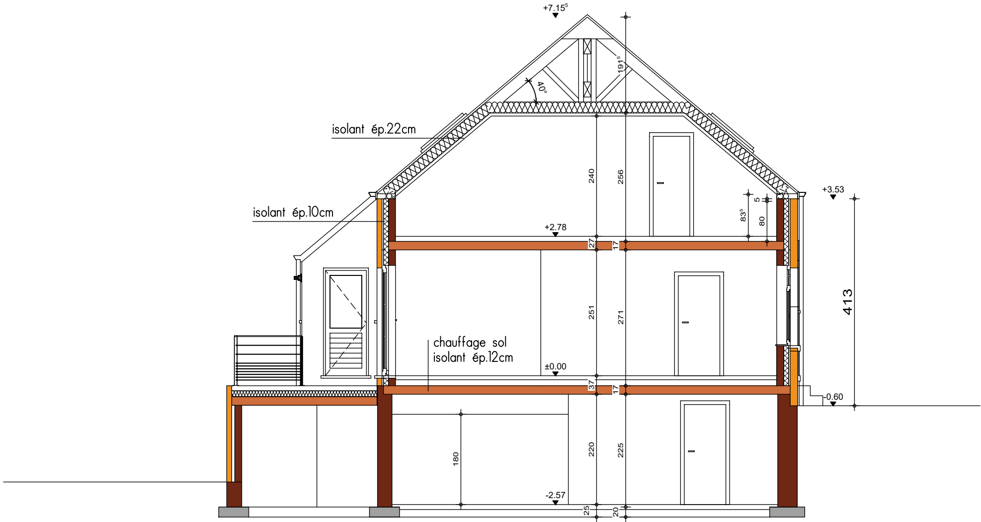
COUPE AA
