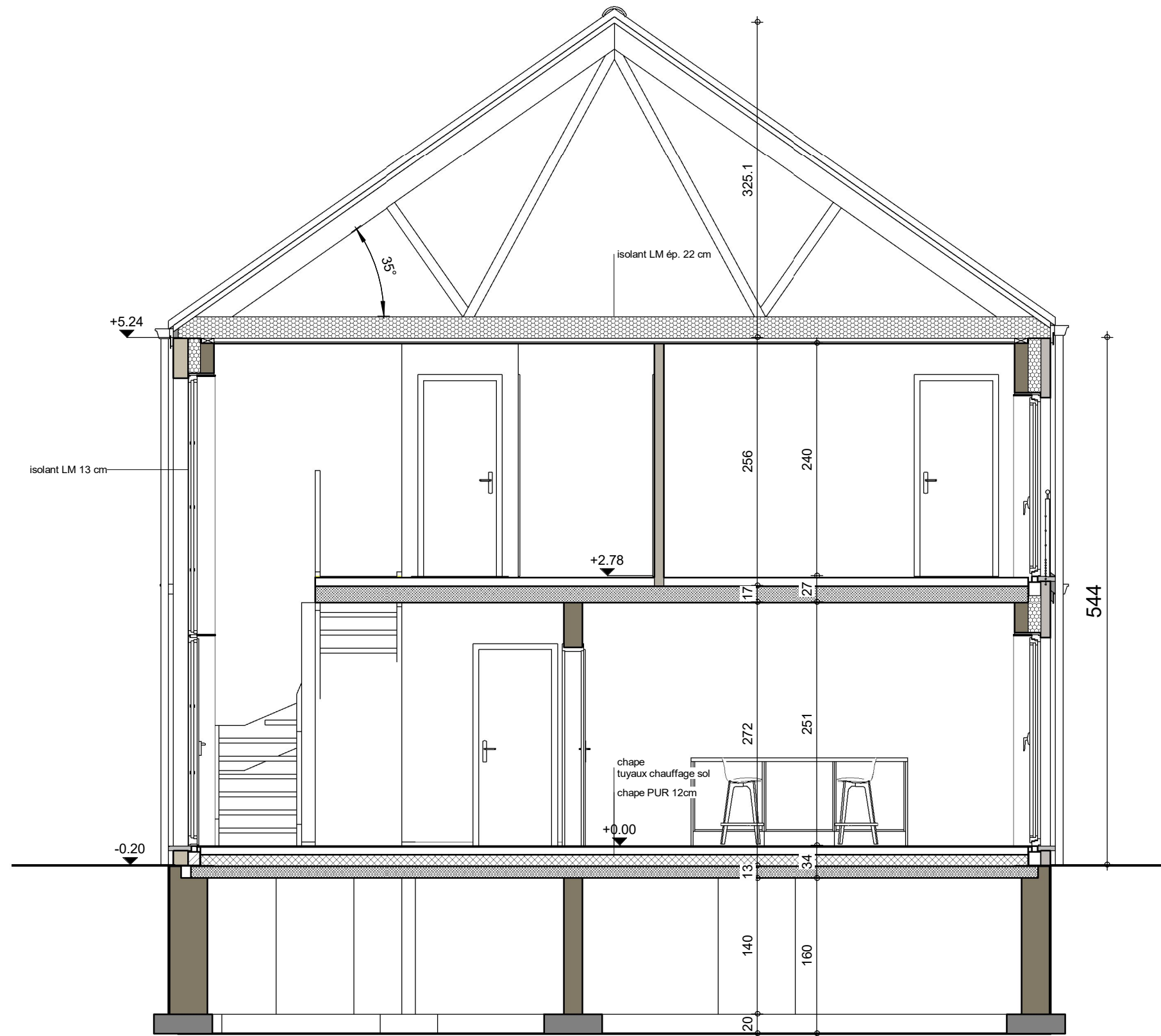
COUPE AA
