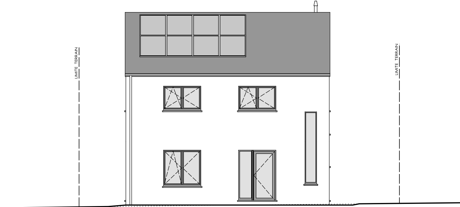
FACADE AVANT
