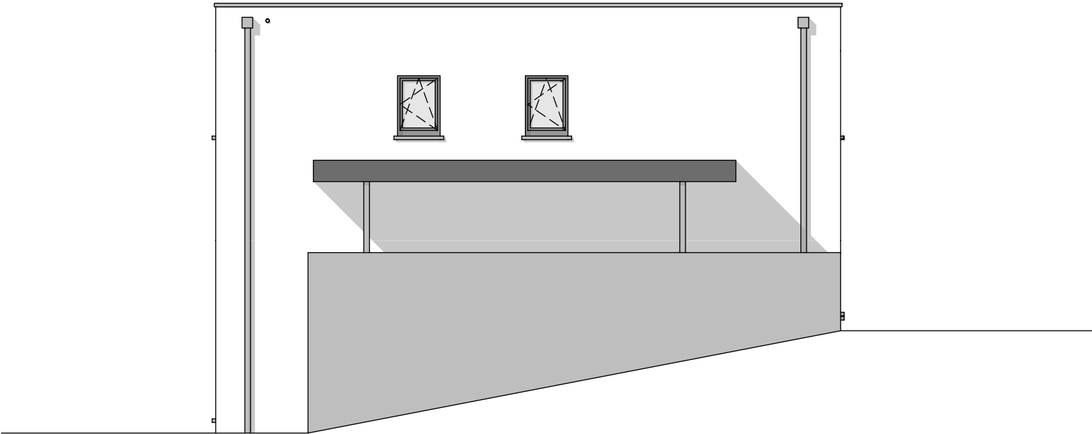
PIGNON GAUCHE
