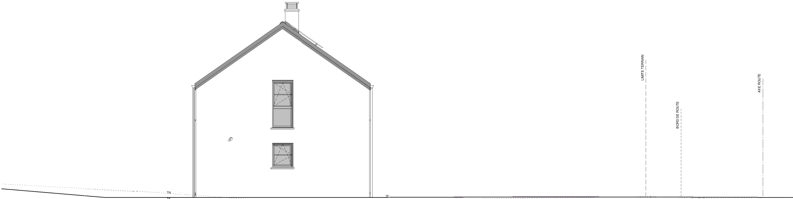
PIGNON GAUCHE
