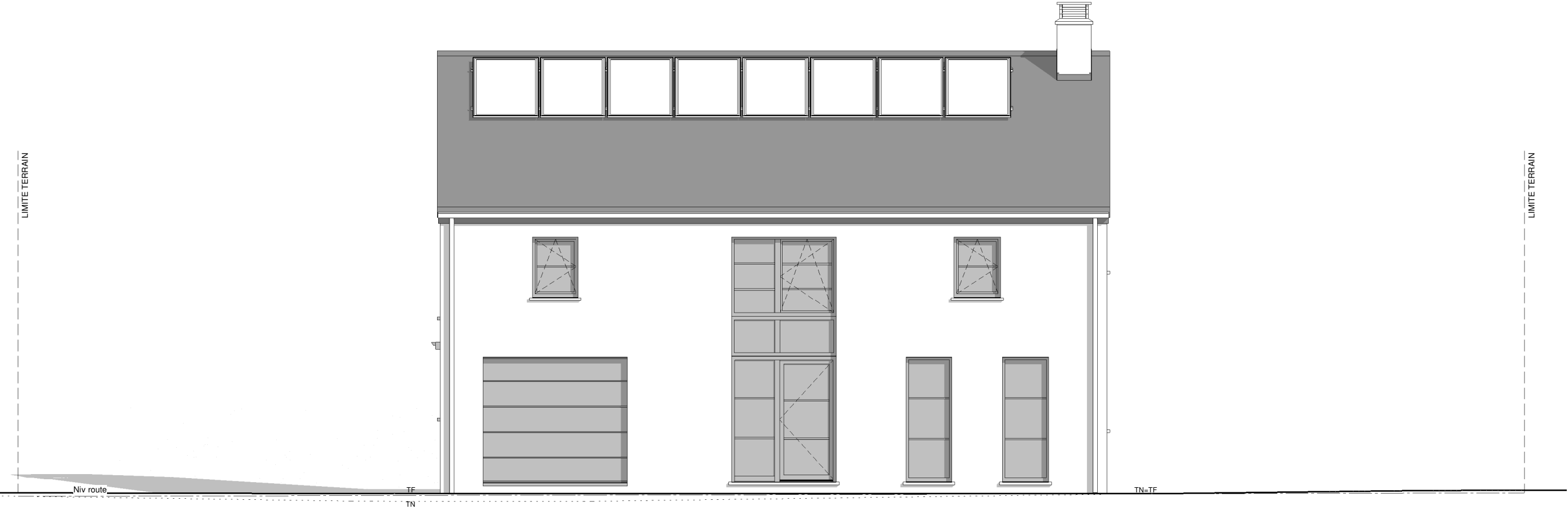
FACADE AVANT
