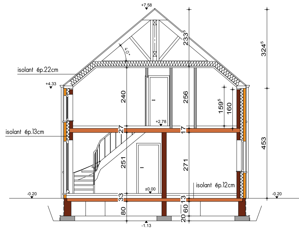
COUPE AA
