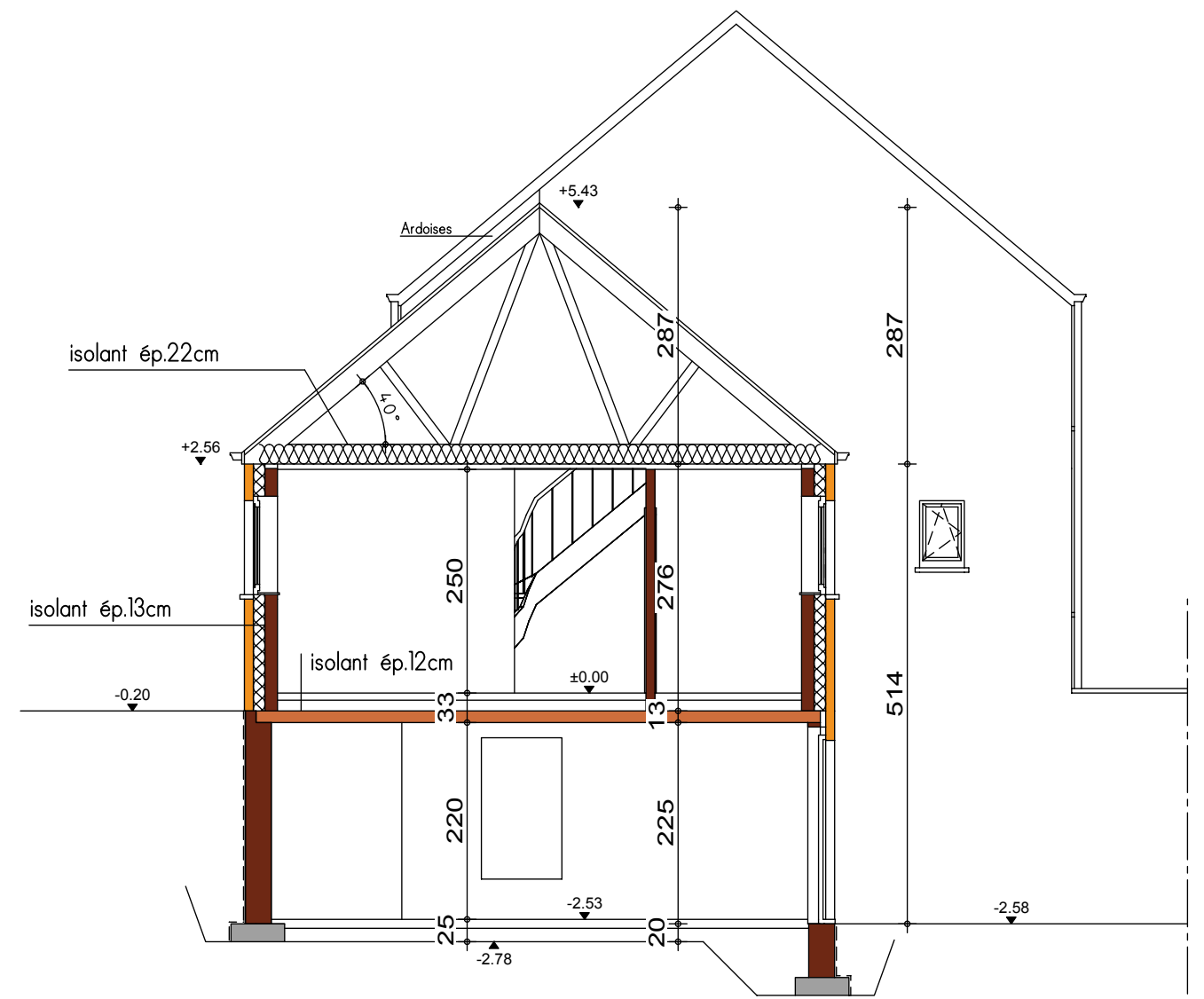
COUPE BB
