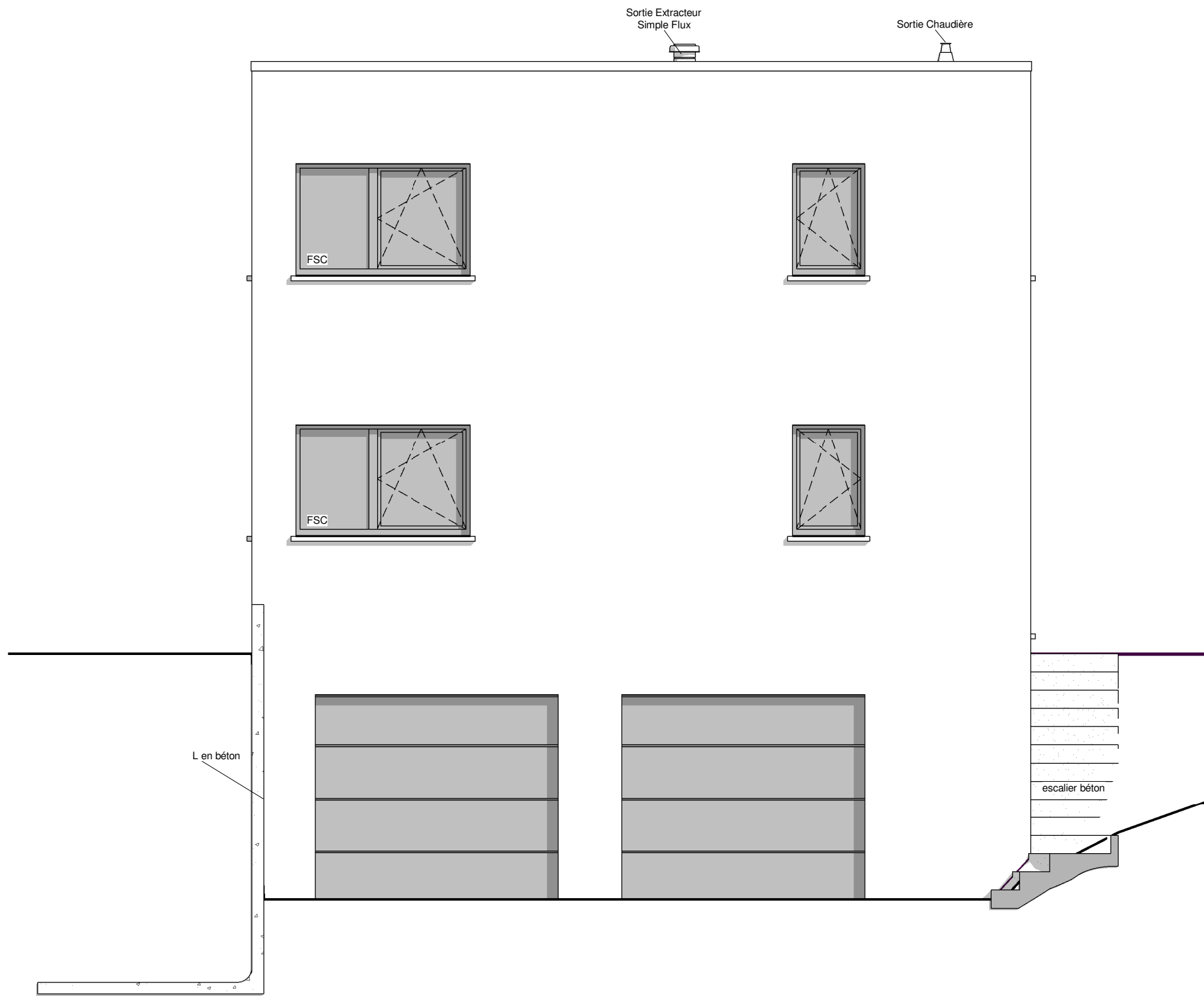
FACADE AVANT
