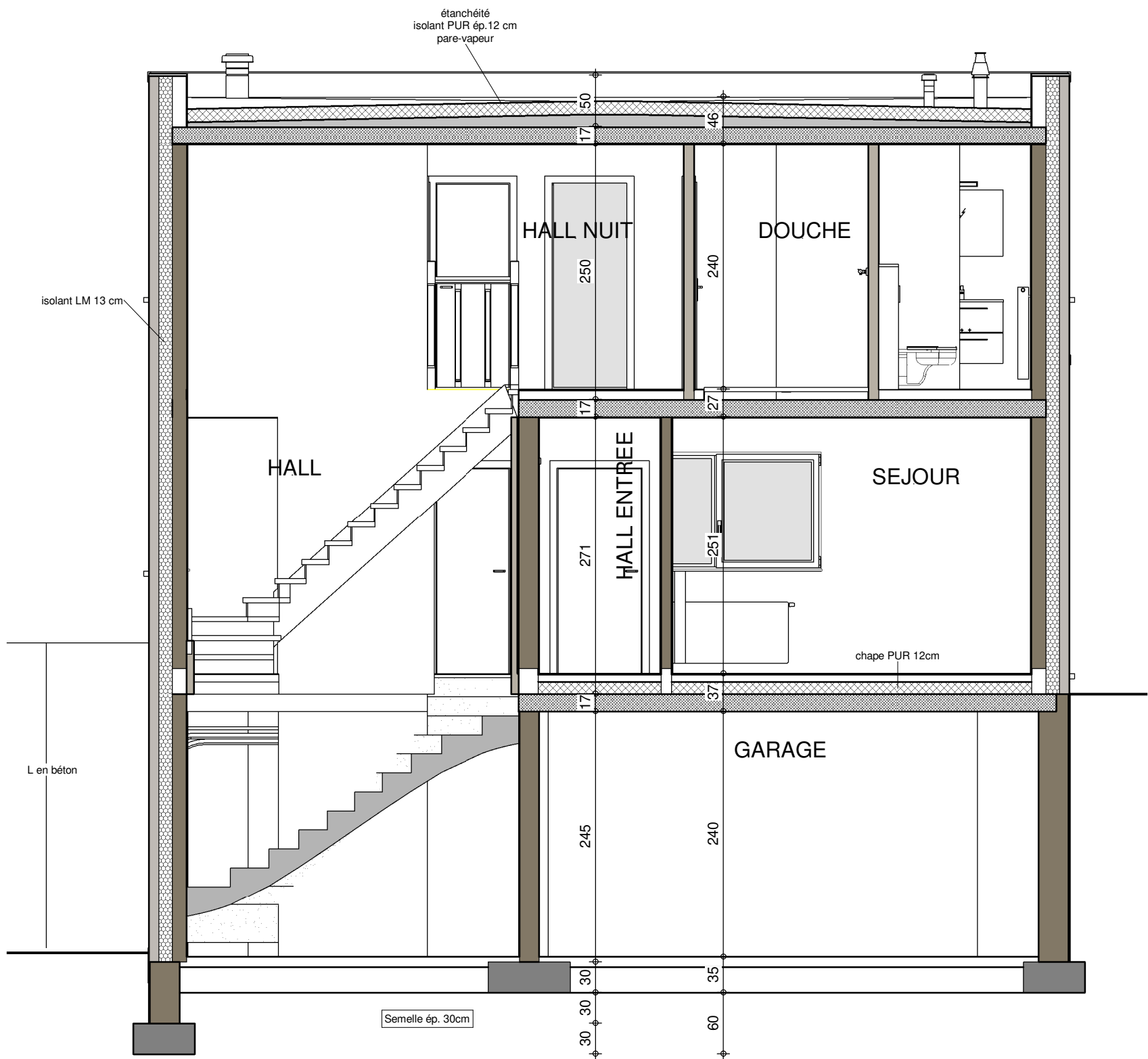
COUPE AA
