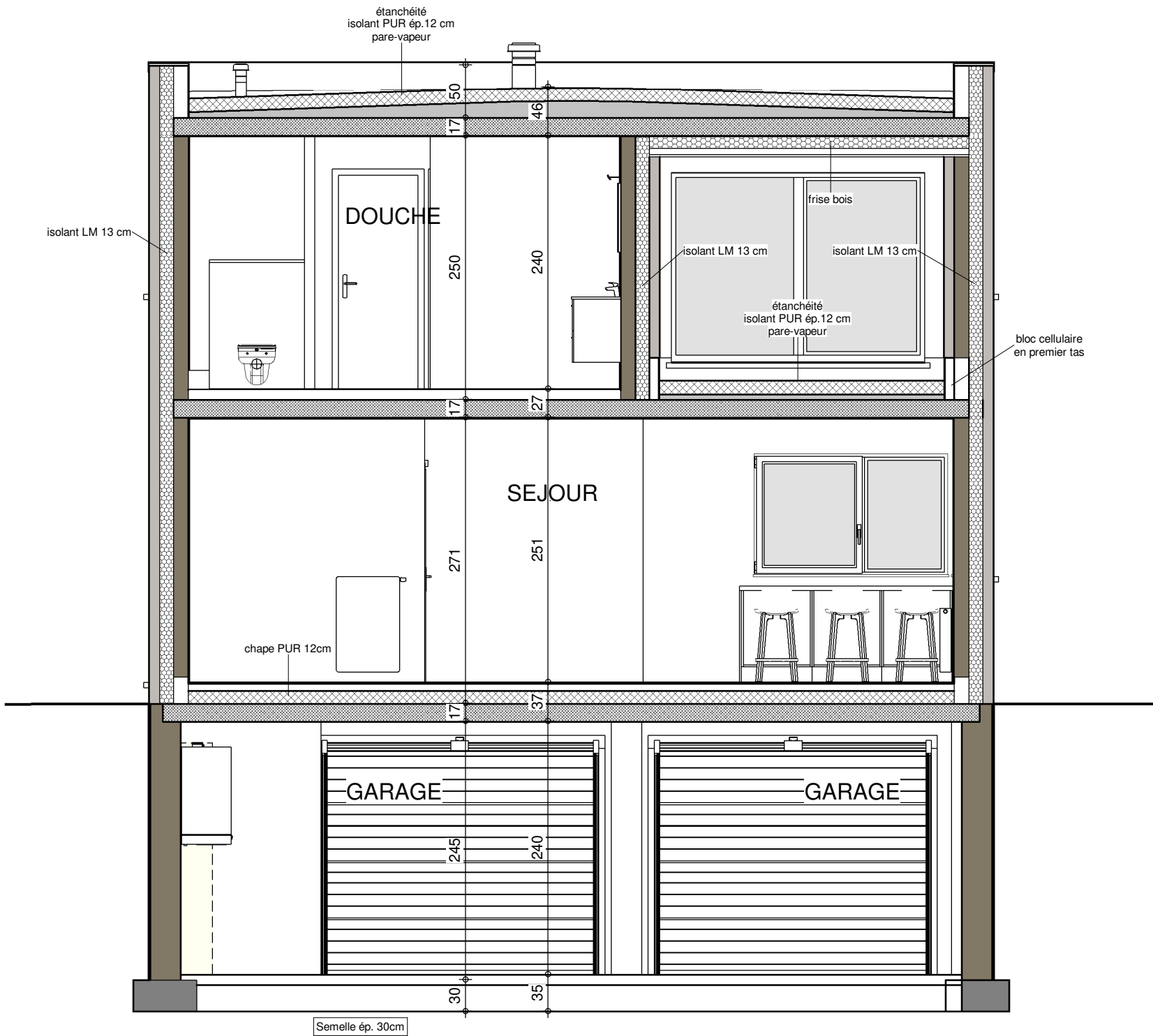
COUPE BB
