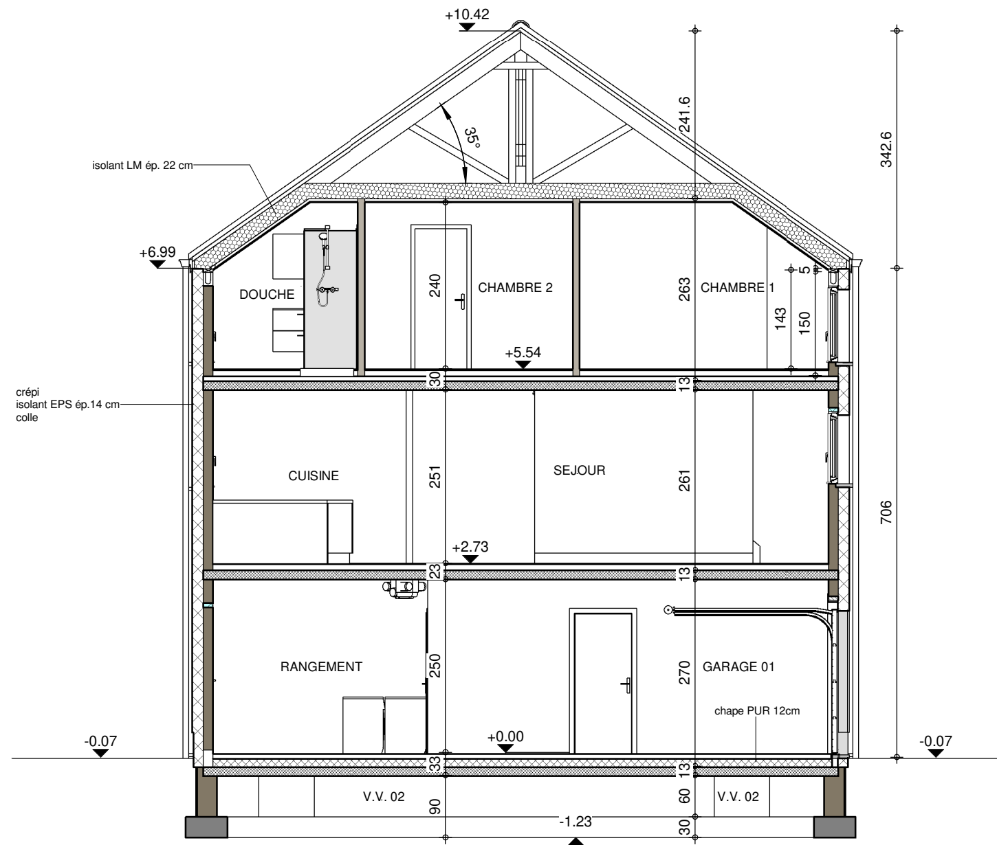
COUPE AA
