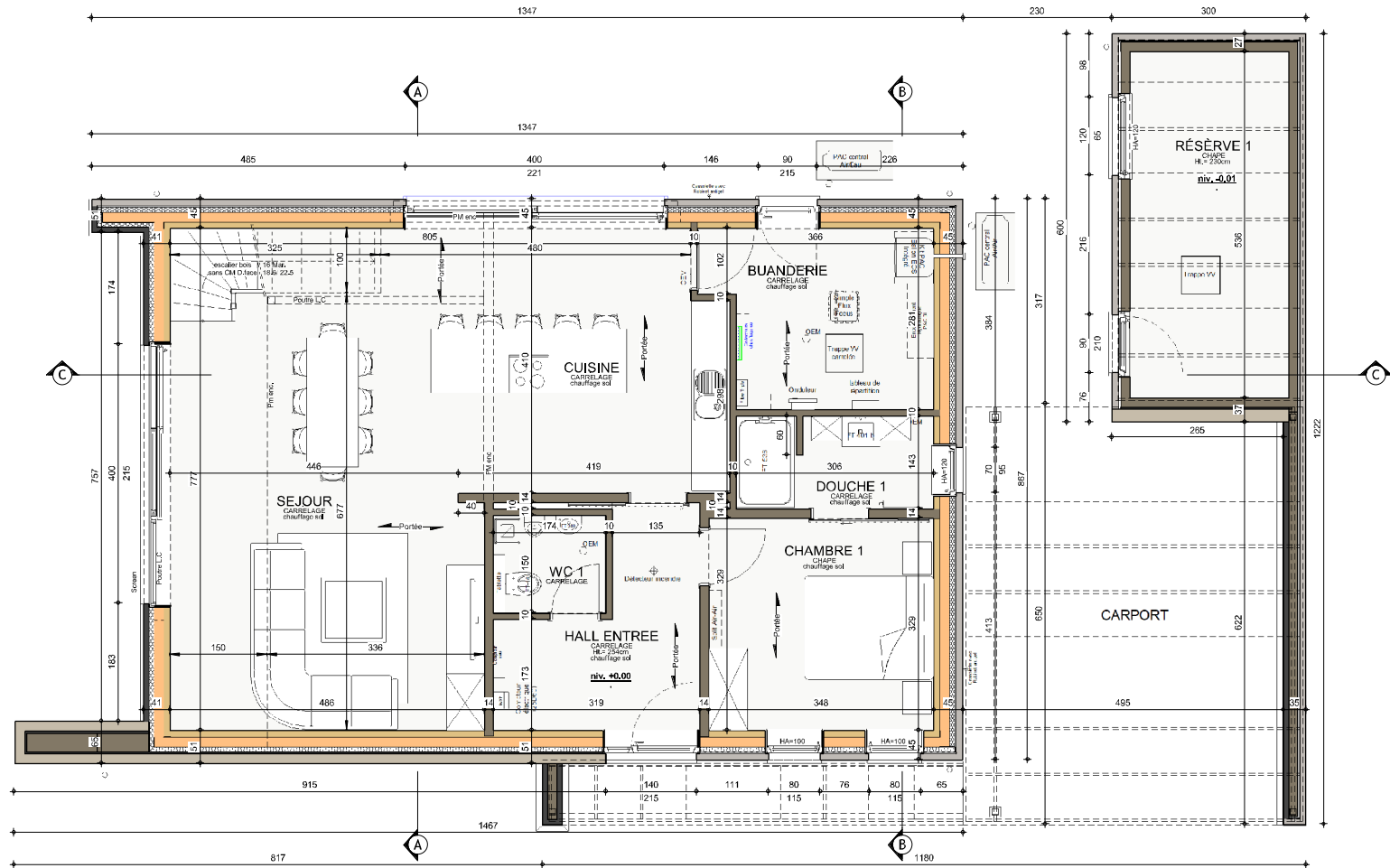
REZ-DE-CHAUSSEE
