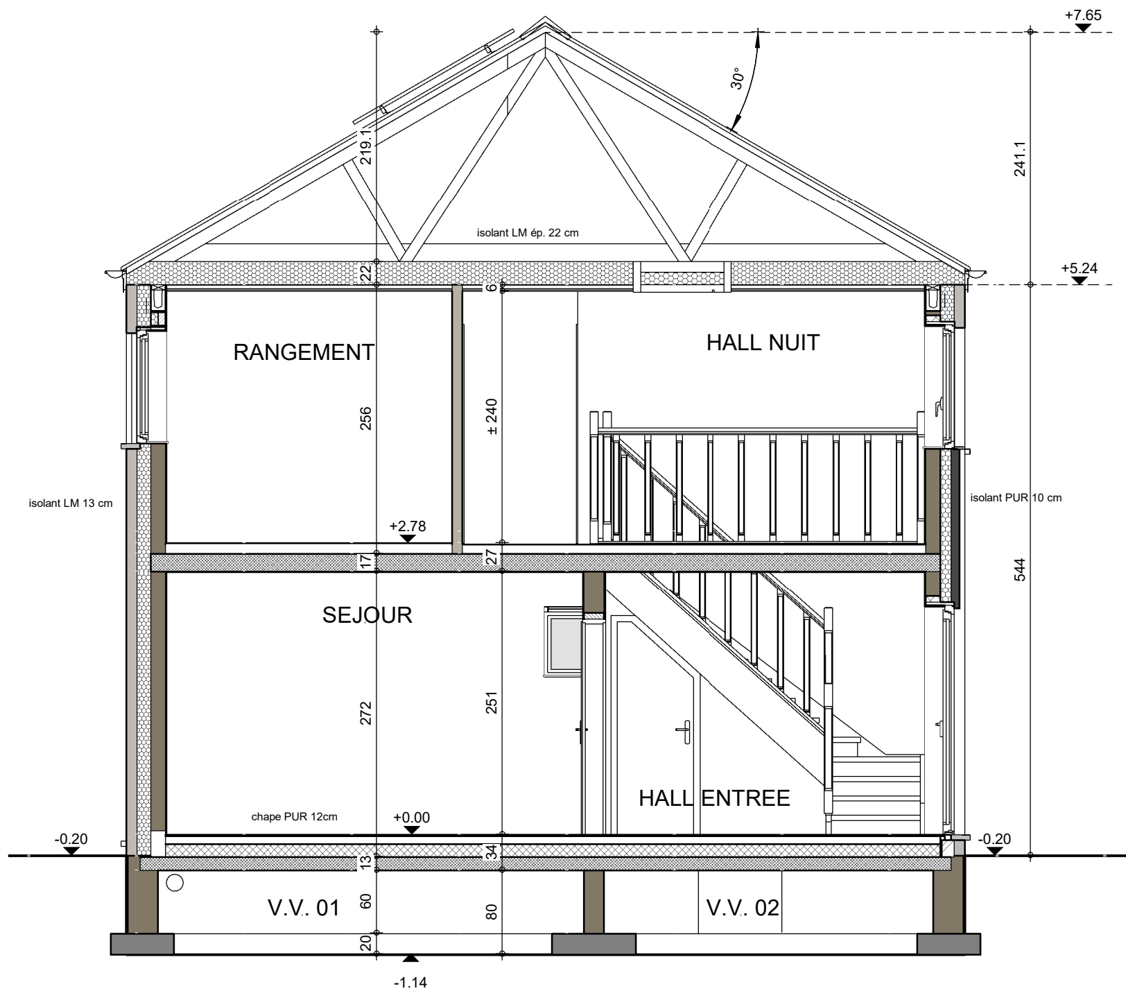
COUPE AA
