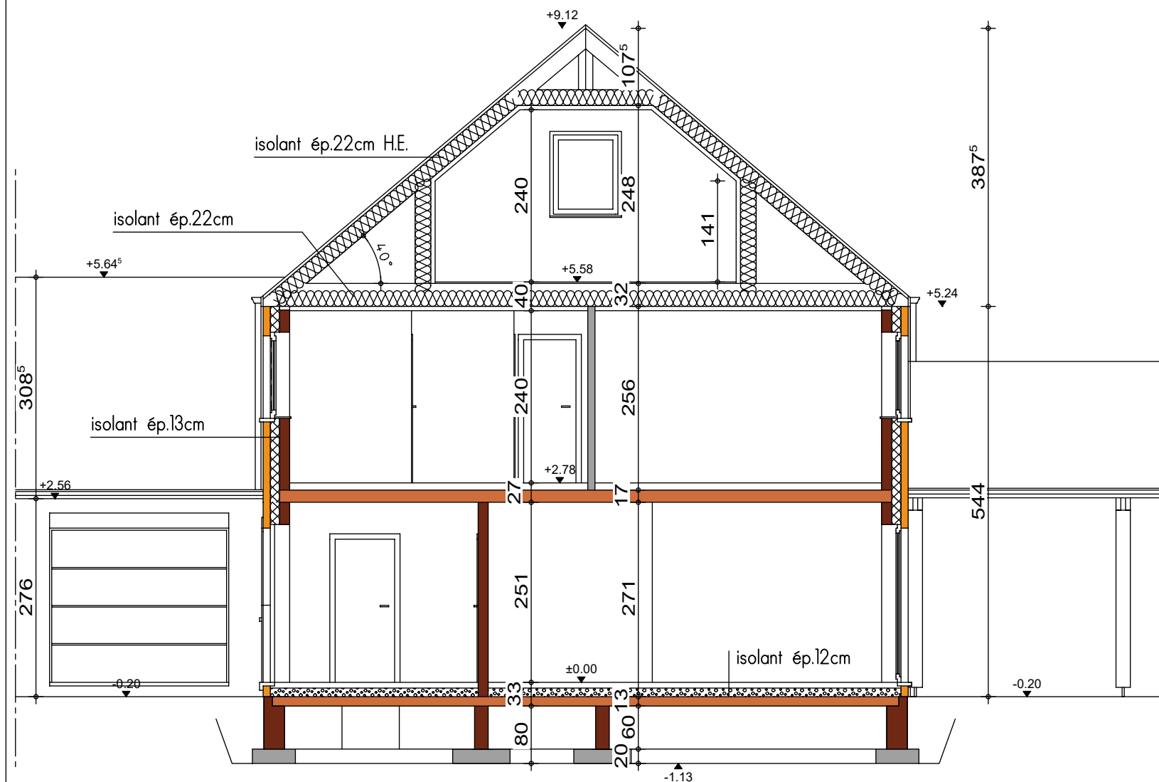
COUPE AA
