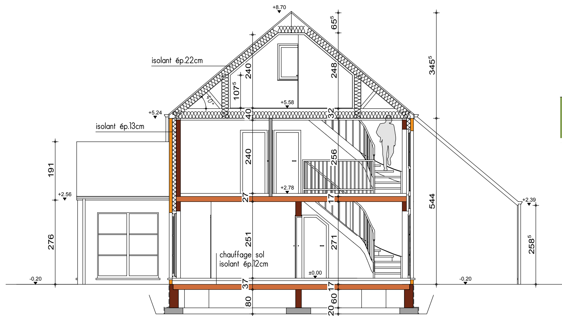
COUPE AA
