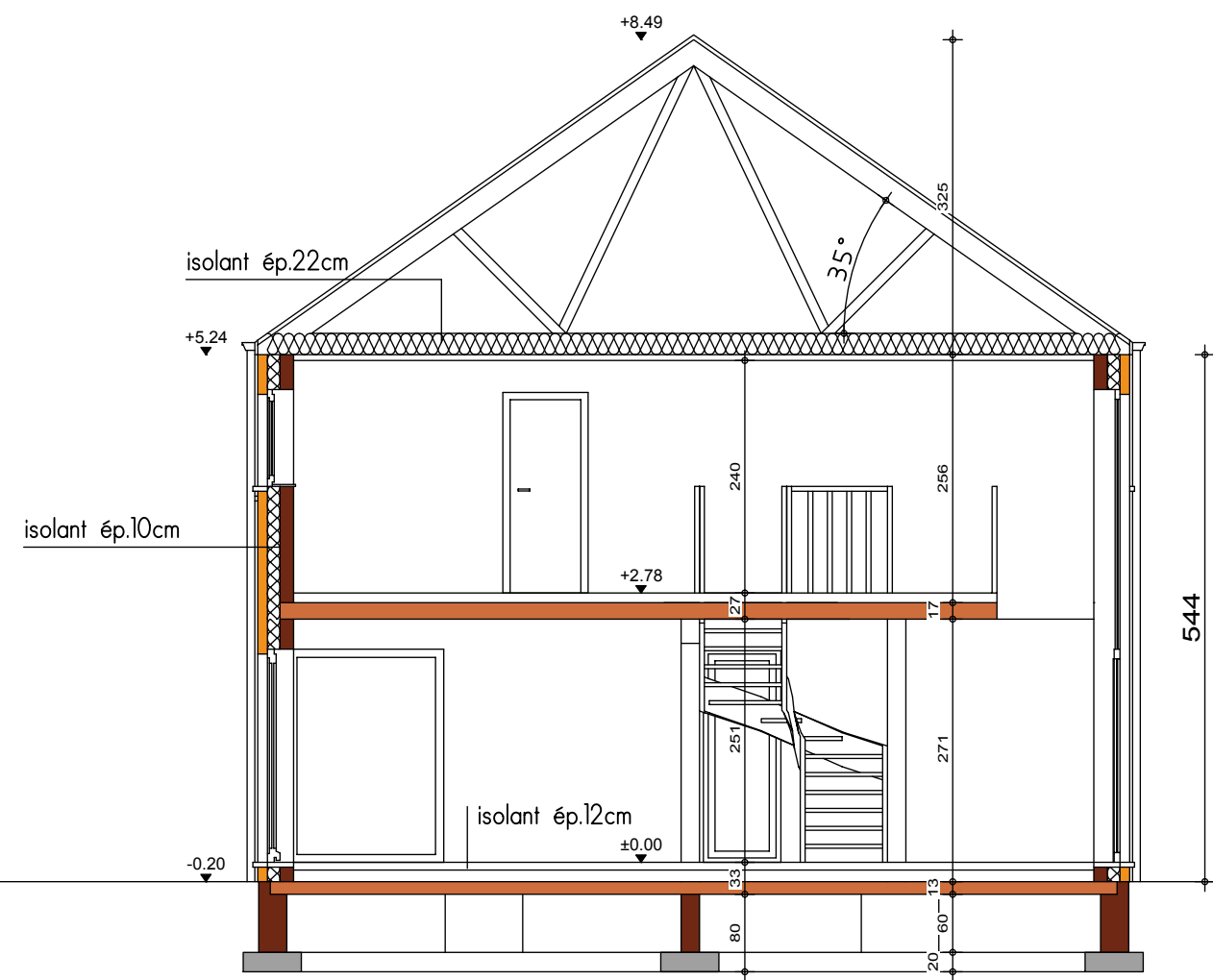
COUPE AA
