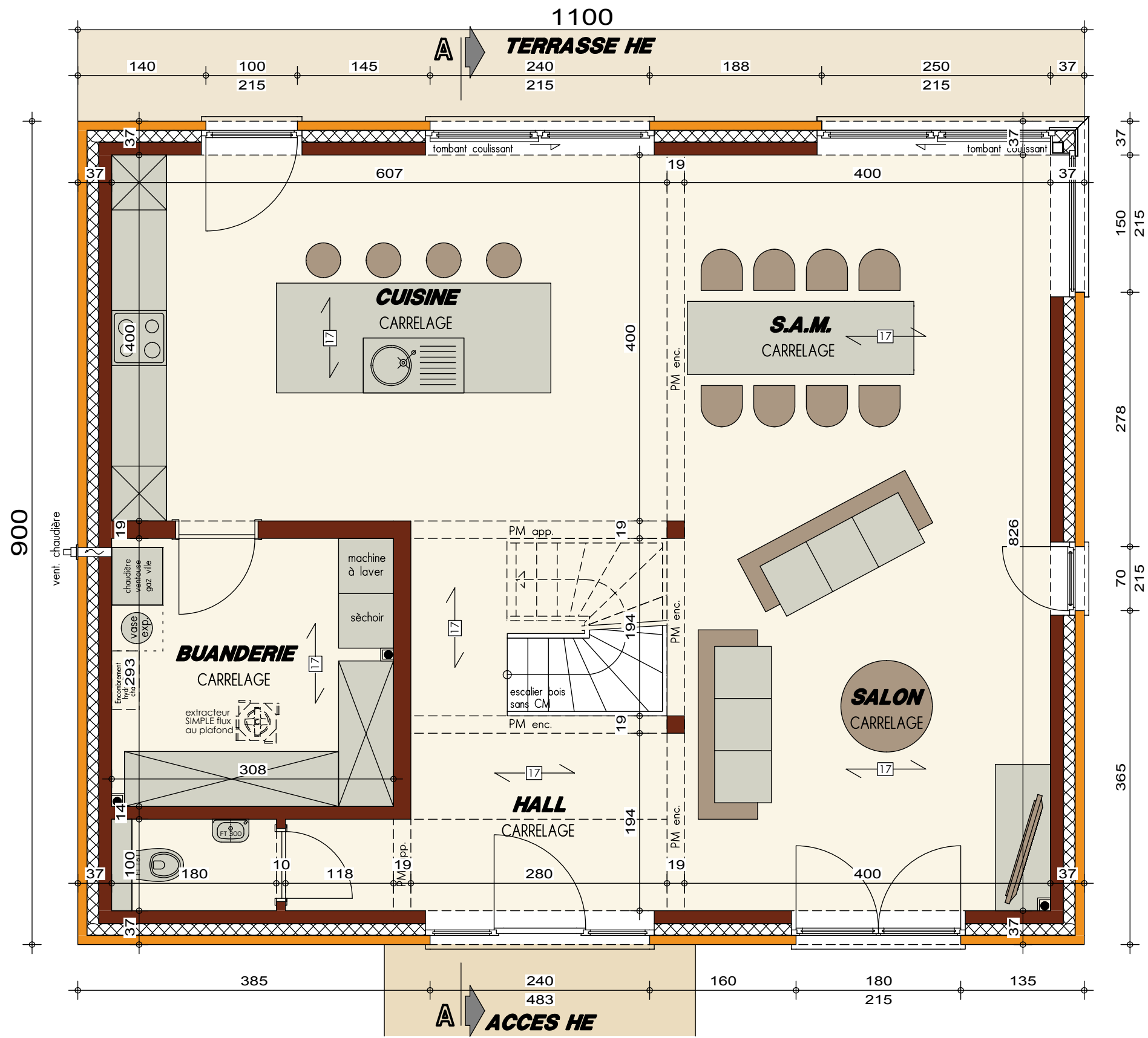
PLAN REZ-DE-CHAUSSEE
