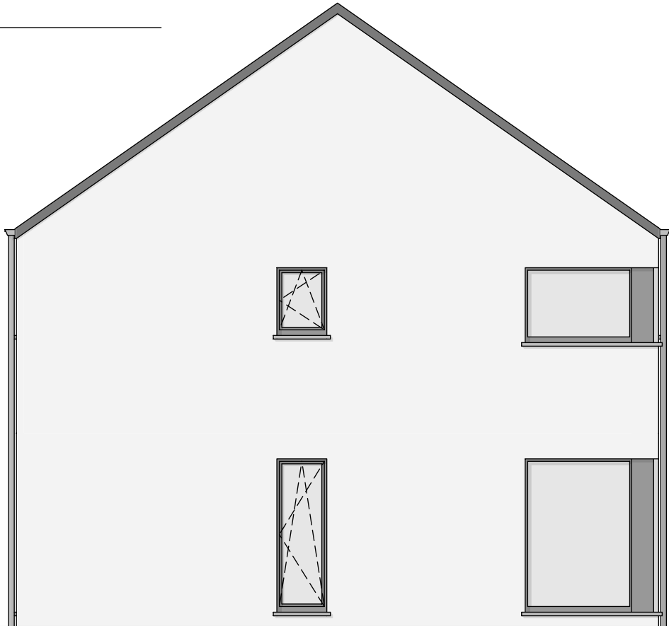
PIGNON DROIT
