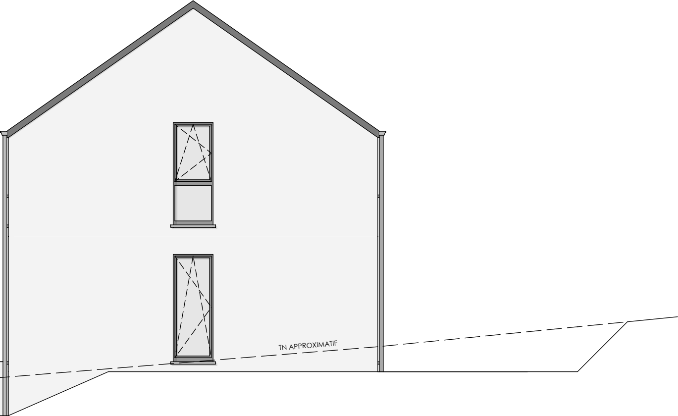
PIGNON DROIT
