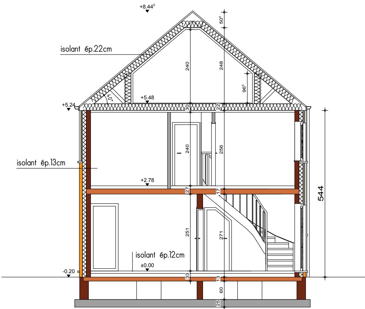
COUPE AA
