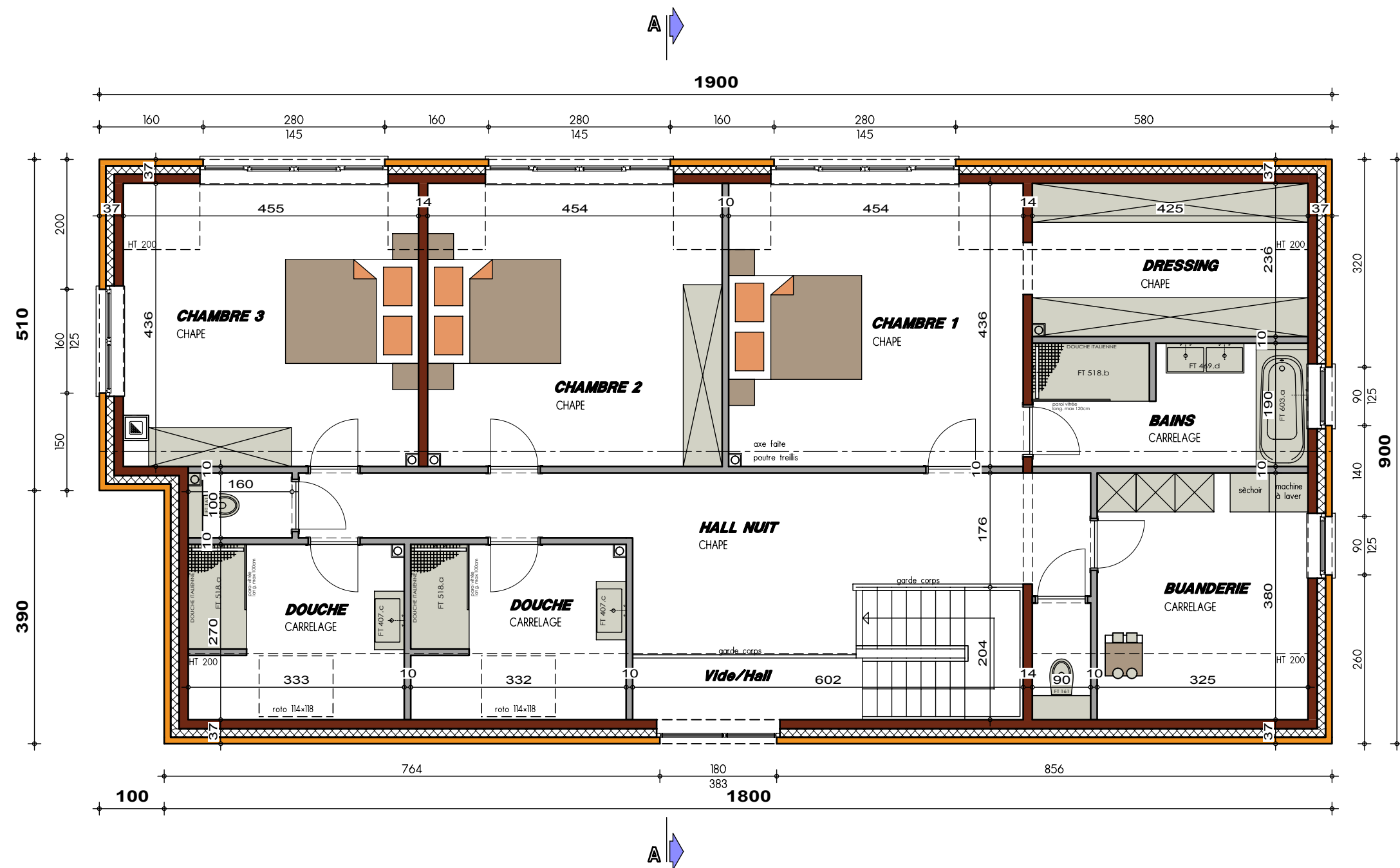
PLAN ETAGE
