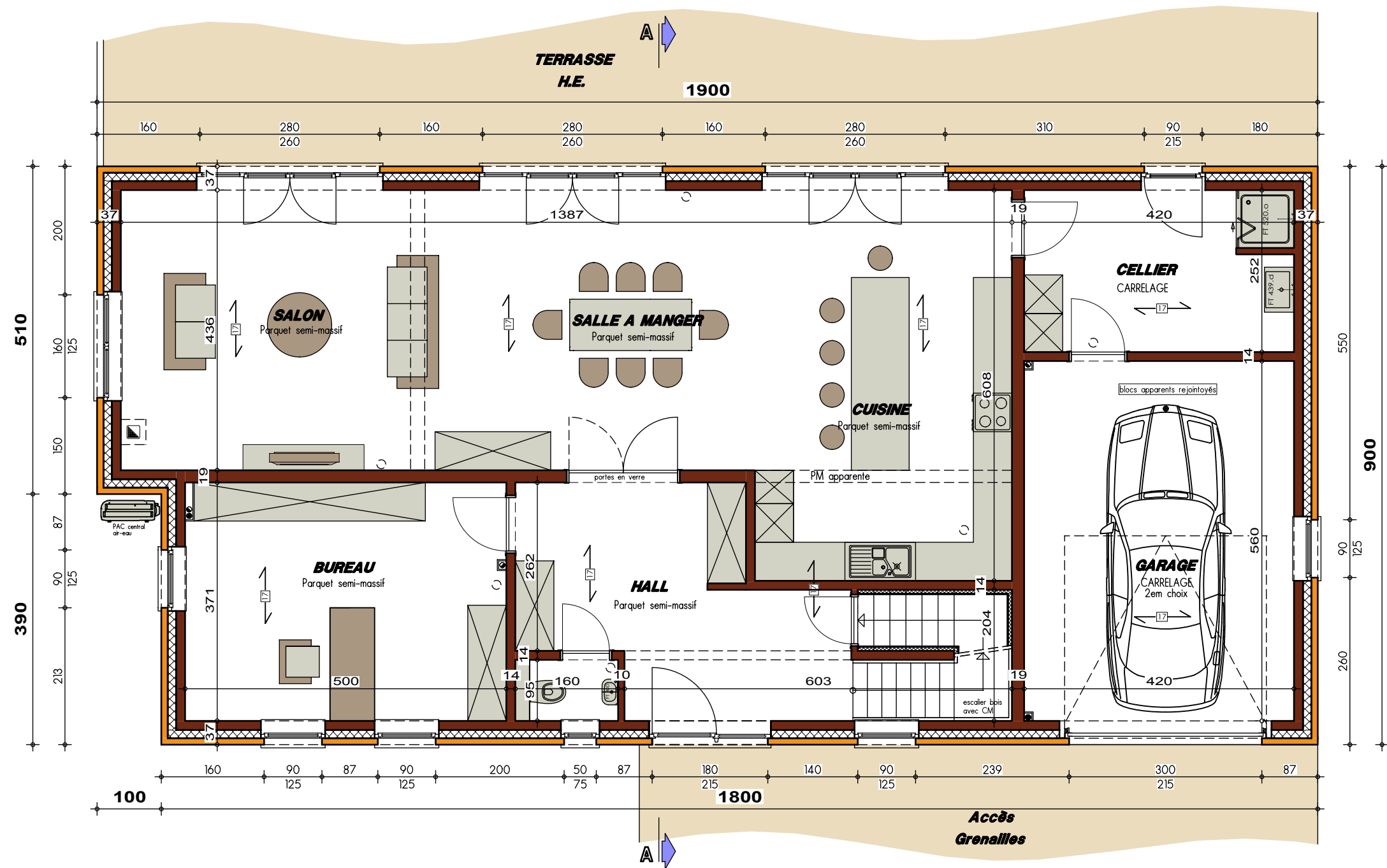
PLAN REZ-DE-CHAUSSEE
