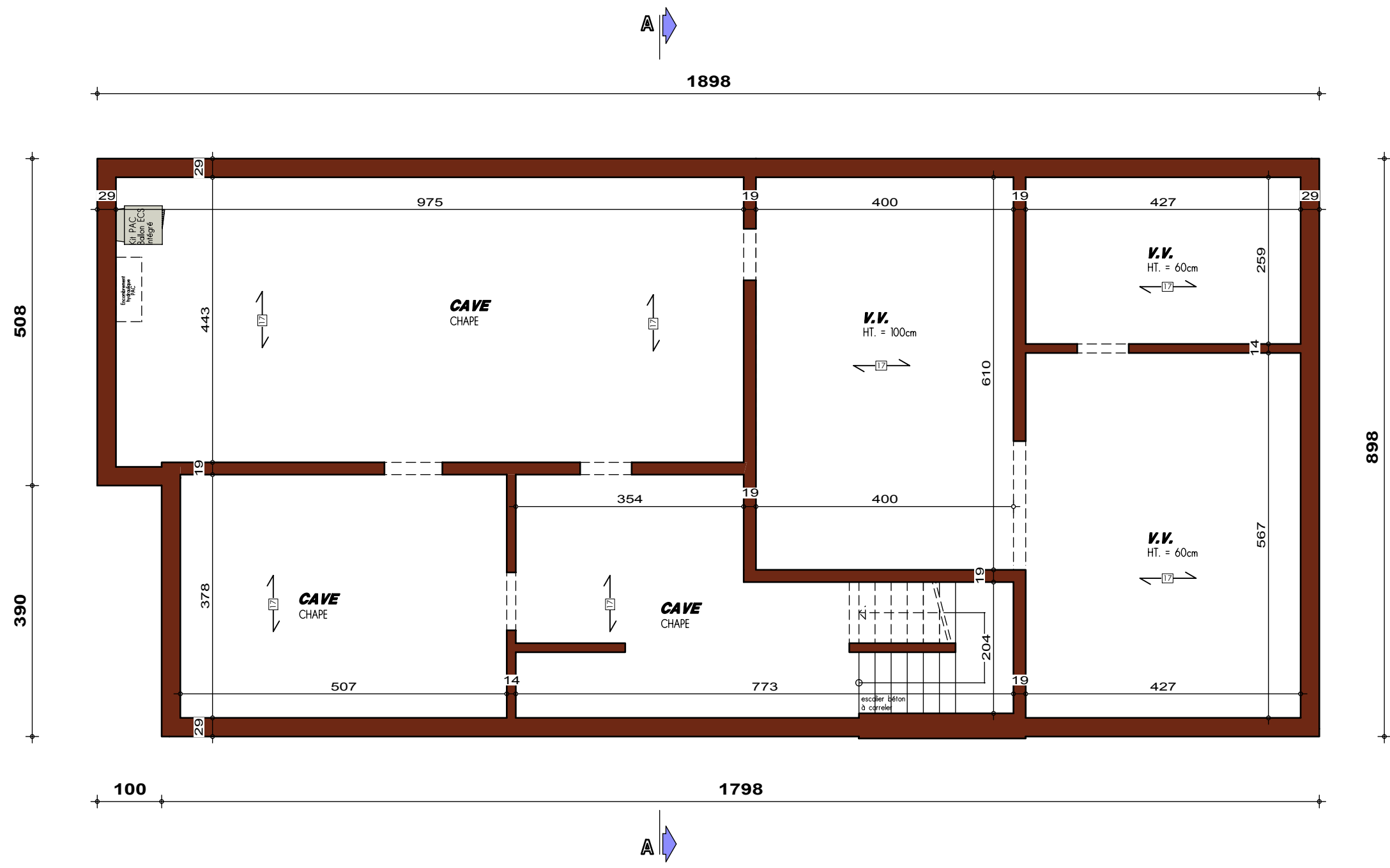
PLAN SOUS-SOL
