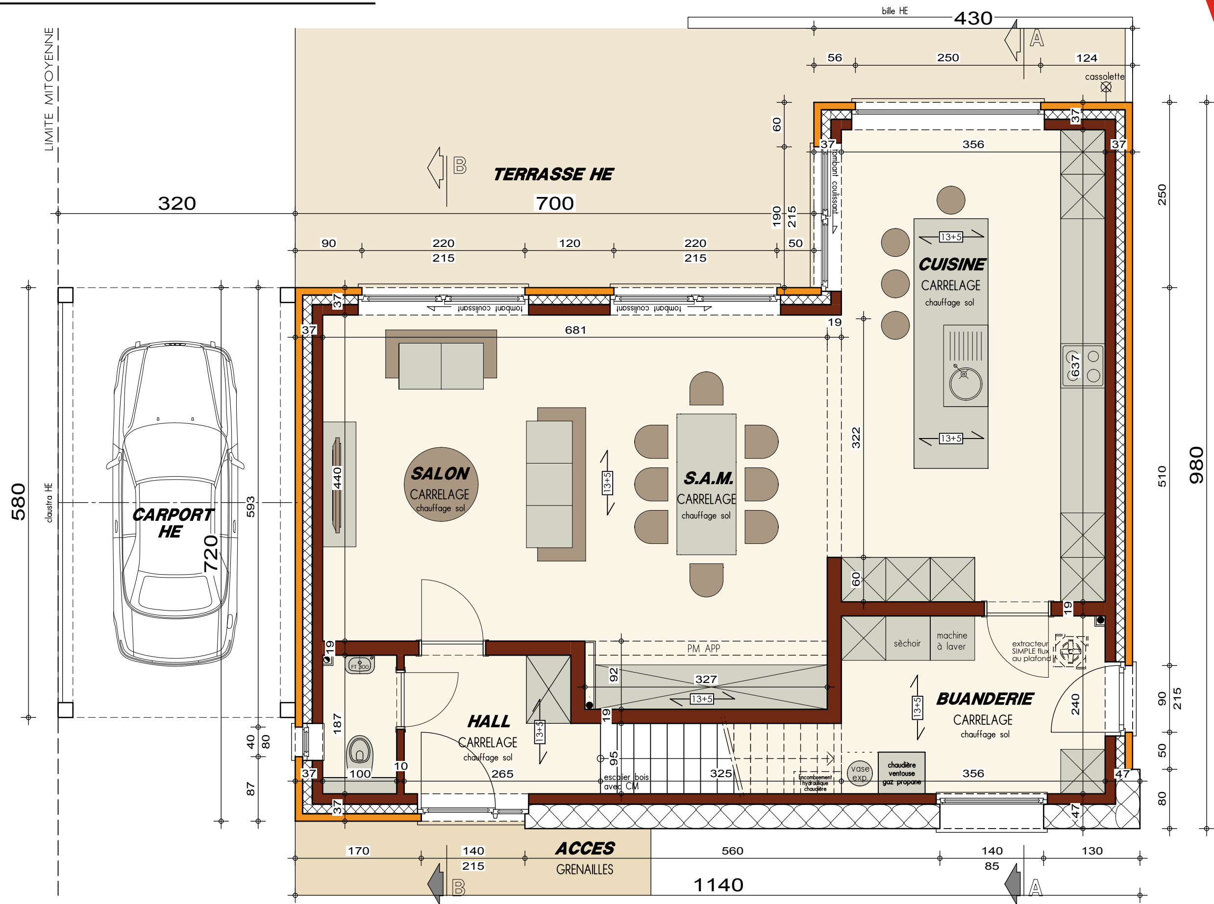
PLAN REZ-DE-CHAUSSEE
