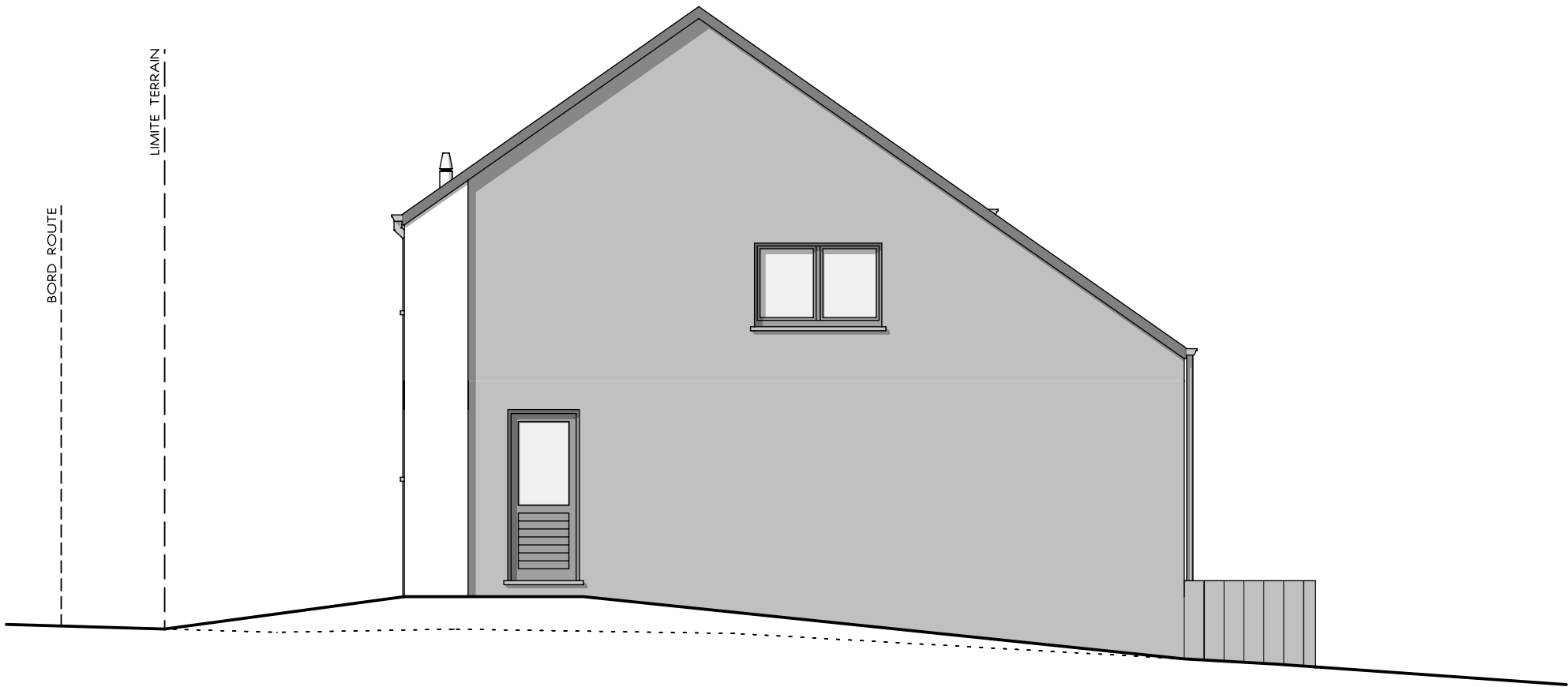
PIGNON DROIT
