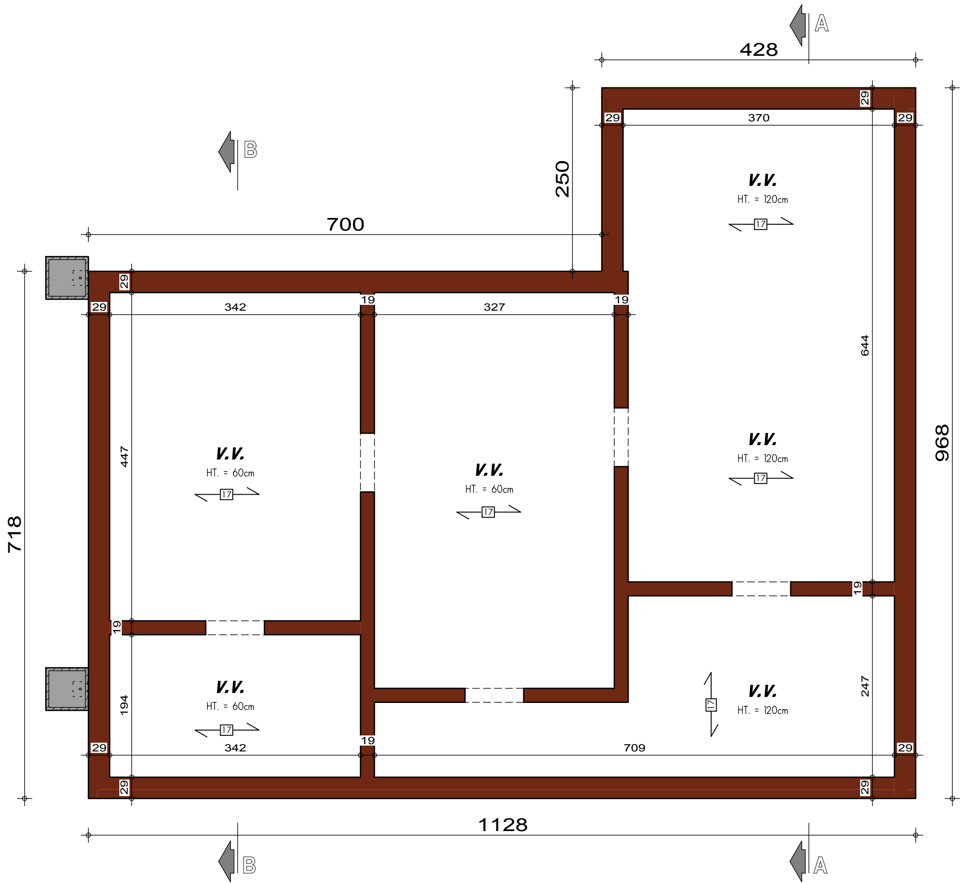
PLAN SOUS-SOL
