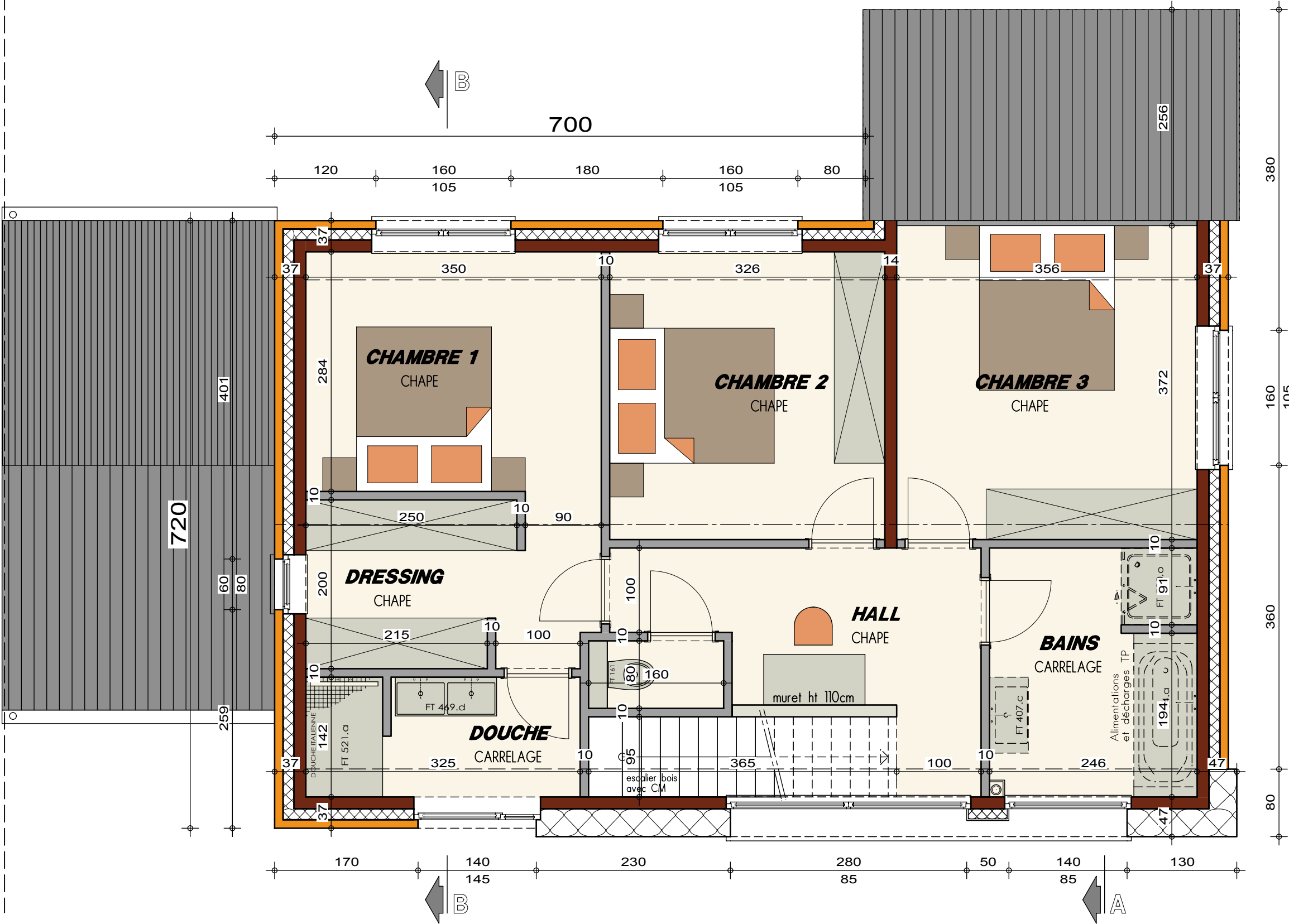
PLAN ETAGE
