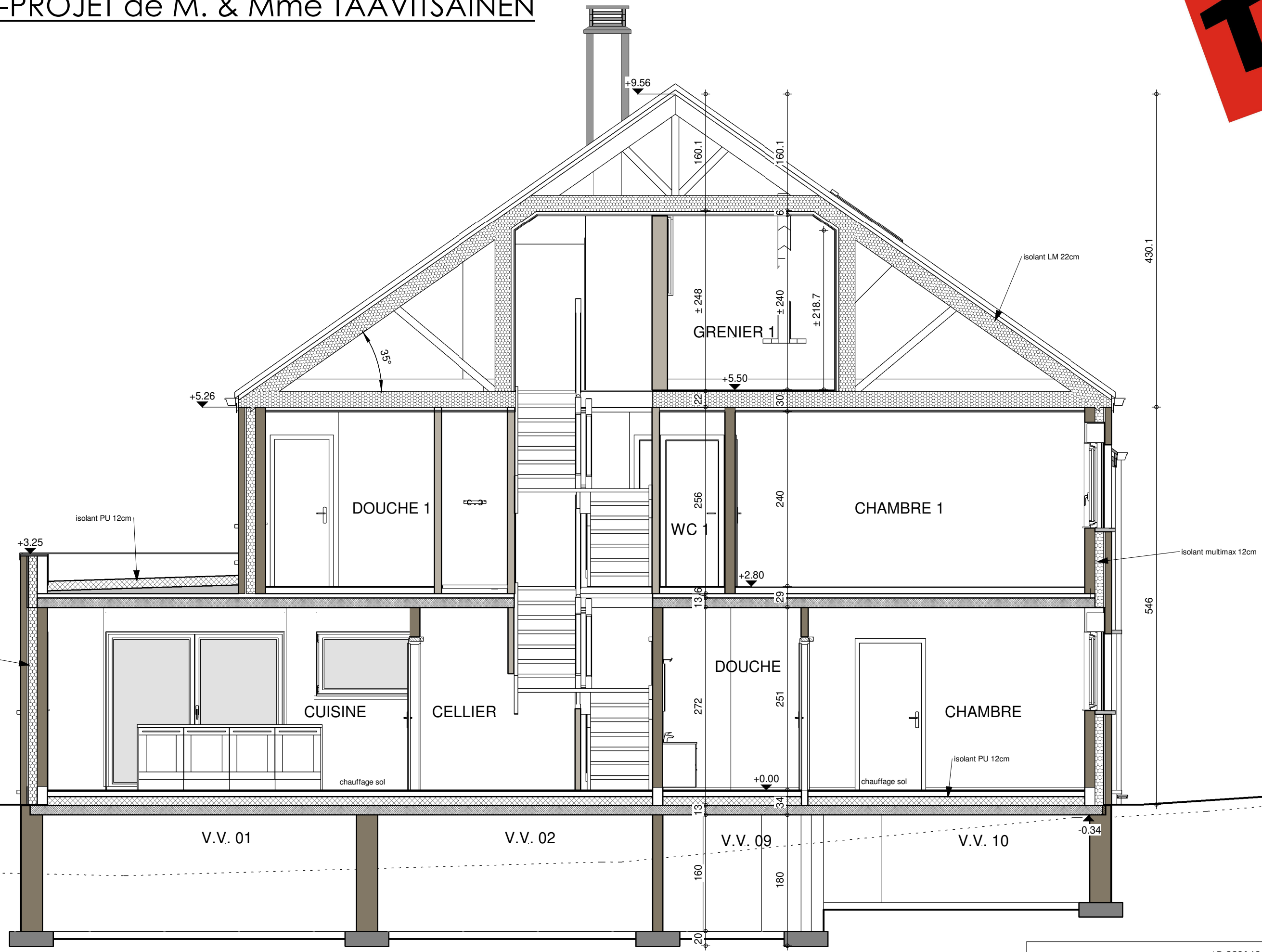
COUPE AA
