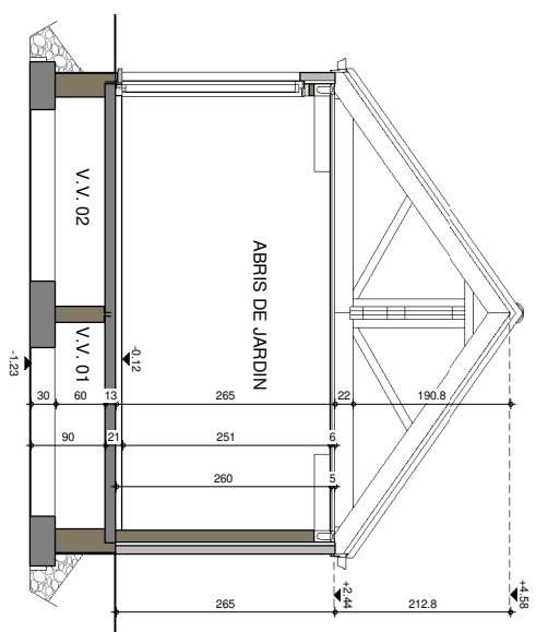
COUPE BB
