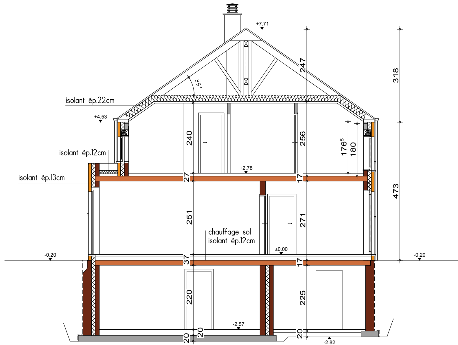
COUPE AA
