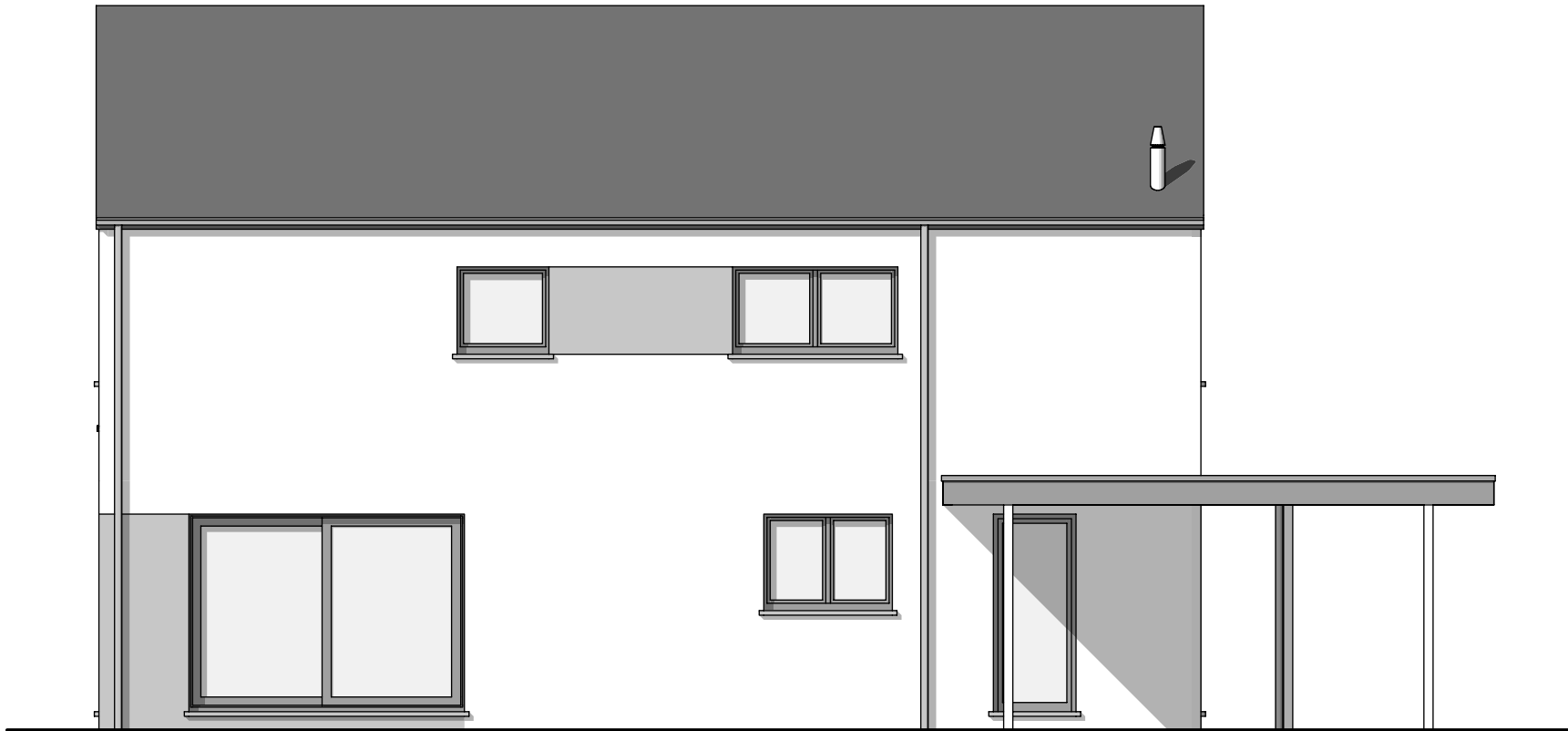
FACADE LATERALE GAUCHE
