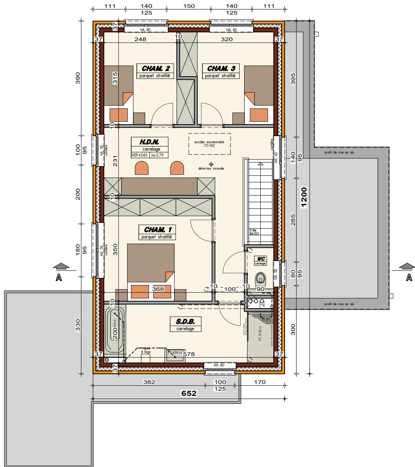
PLAN ETAGE
