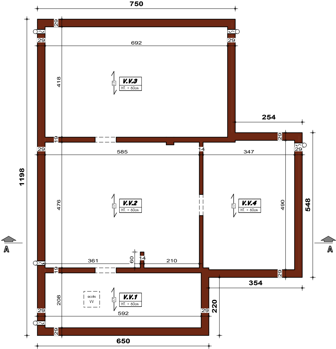
PLAN SOUS-SOL
