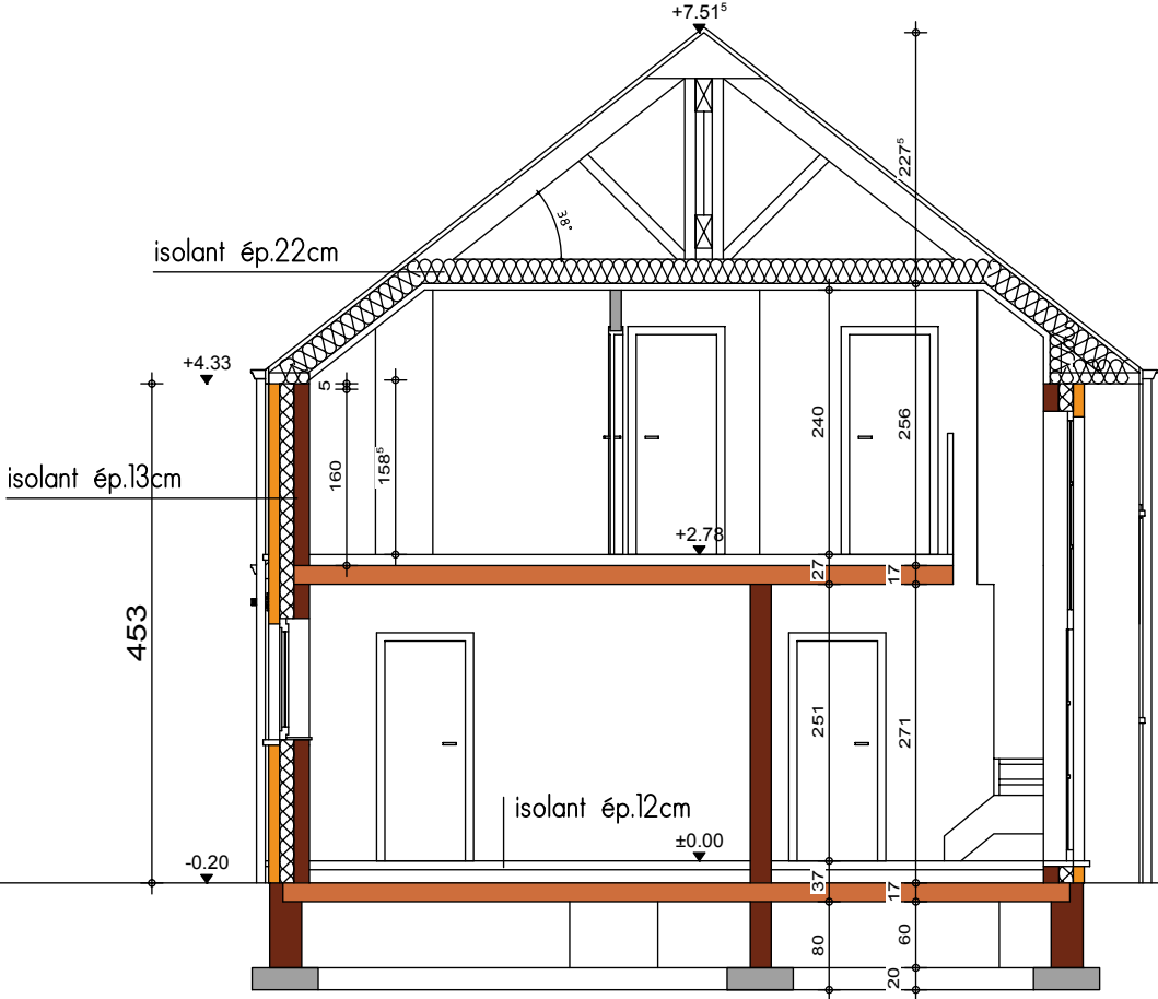
COUPE AA
