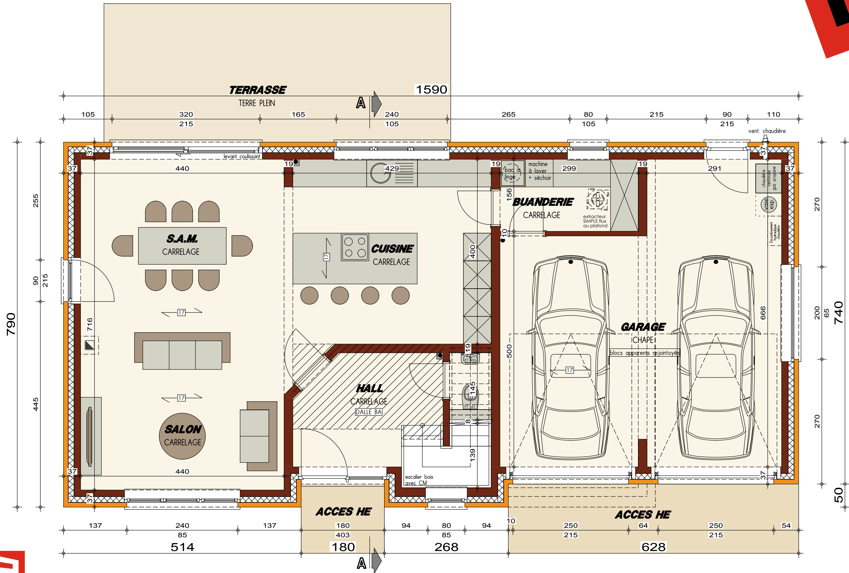
PLAN REZ-DE-CHAUSSEE
