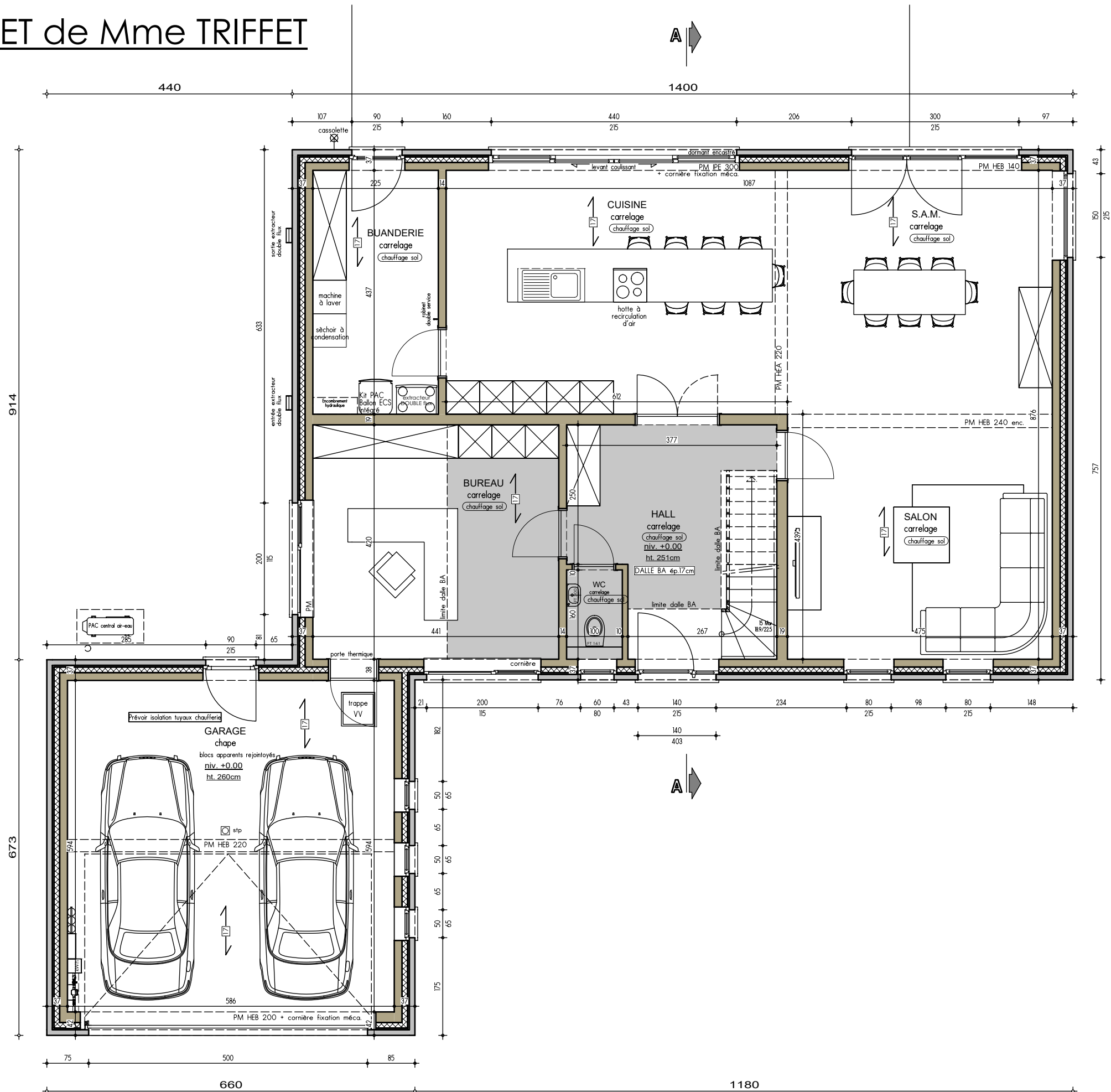
PLAN REZ-DE-CHAUSSEE
