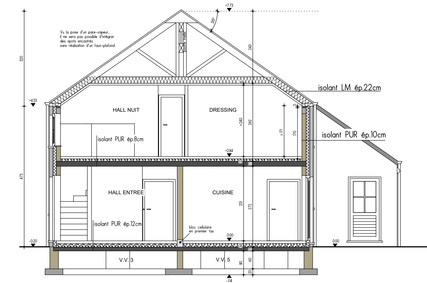
COUPE AA
