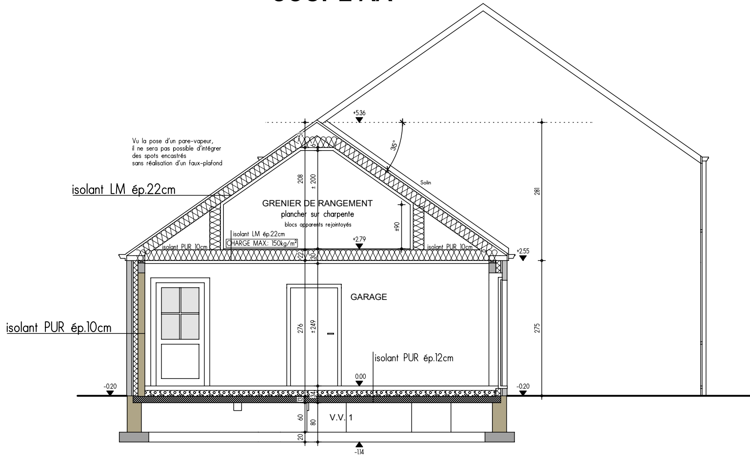
COUPE BB
