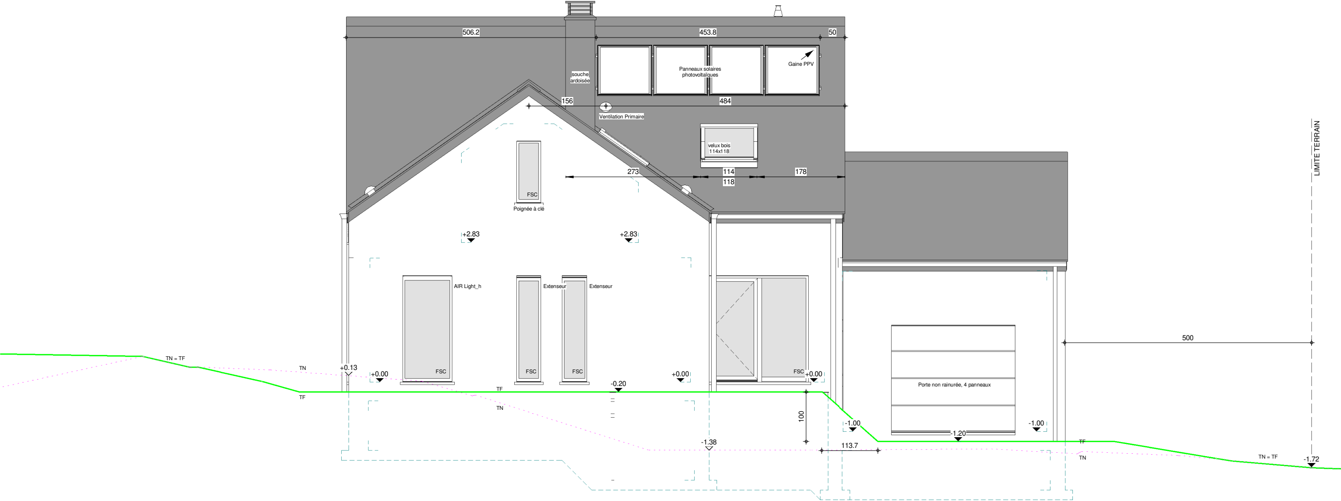
FACADE AVANT
