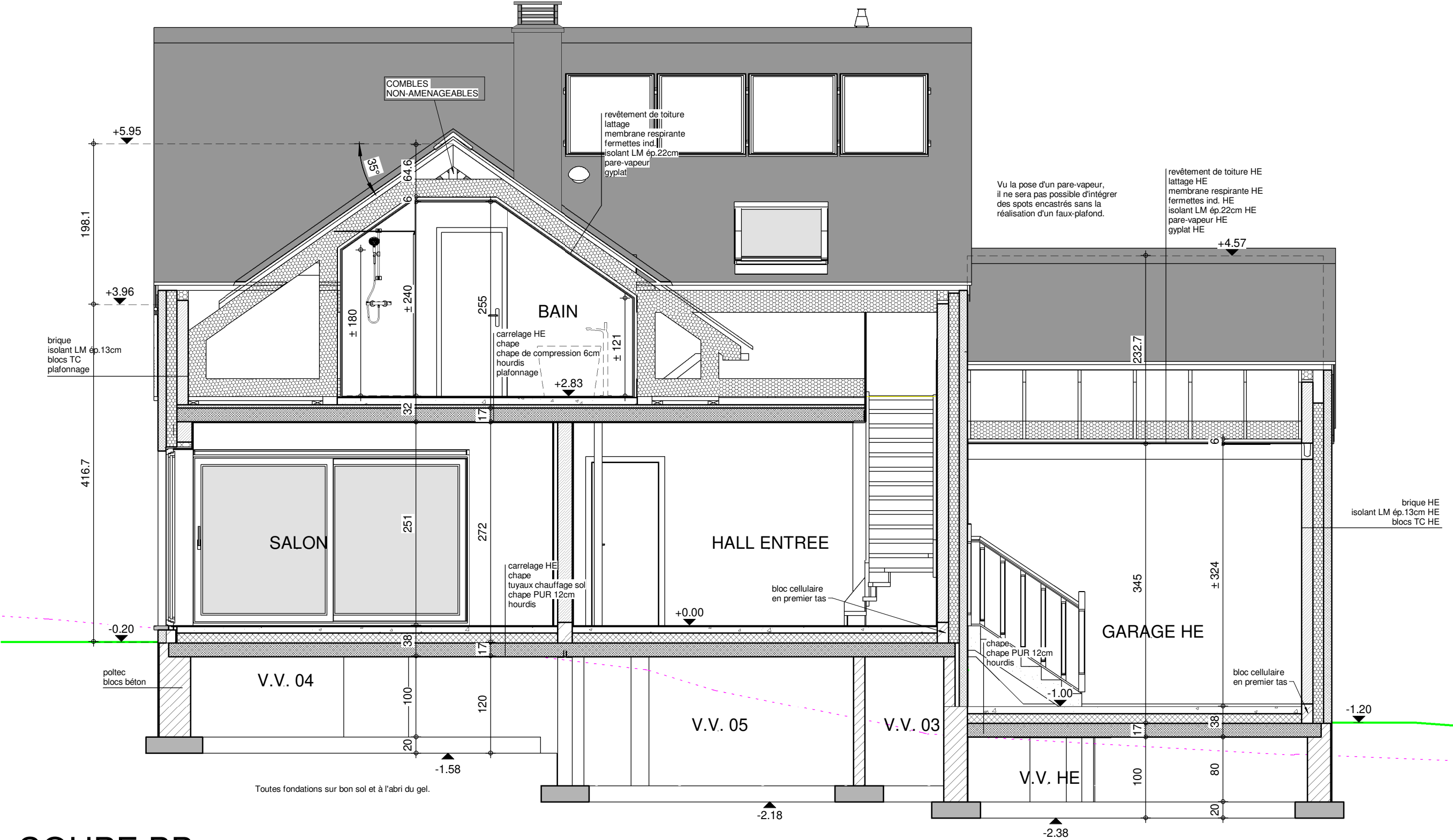
COUPE BB
