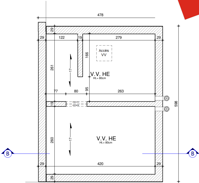
SOUS-SOL - Garage
