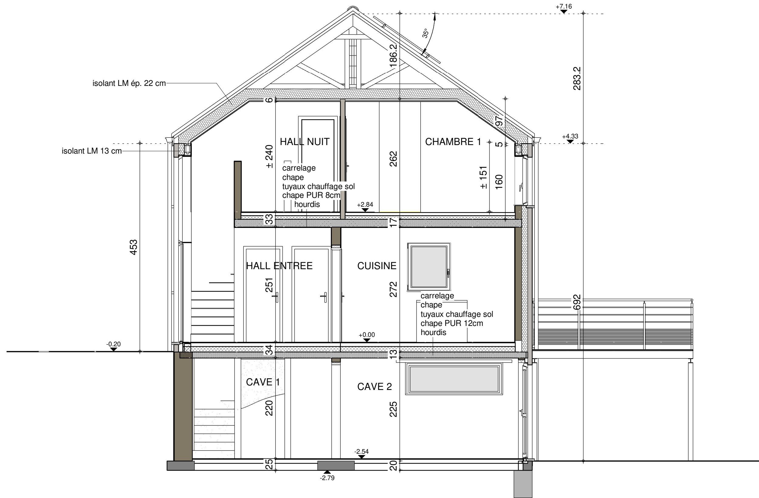
COUPE AA
