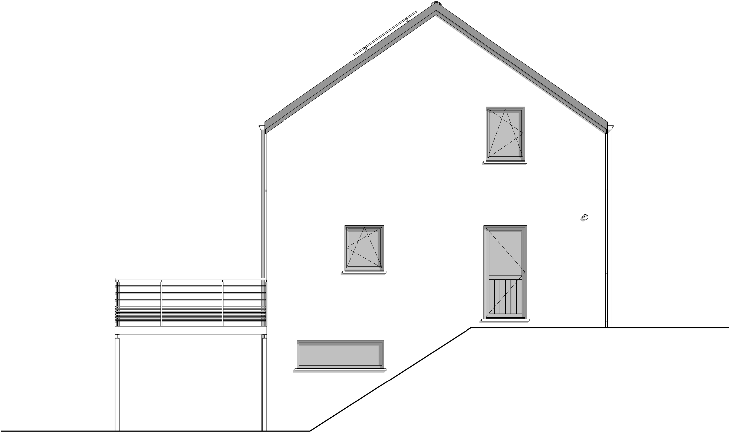
PIGNON GAUCHE
