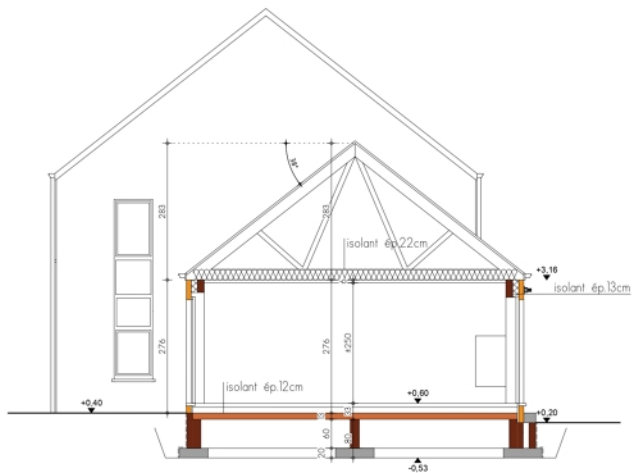
COUPE BB
