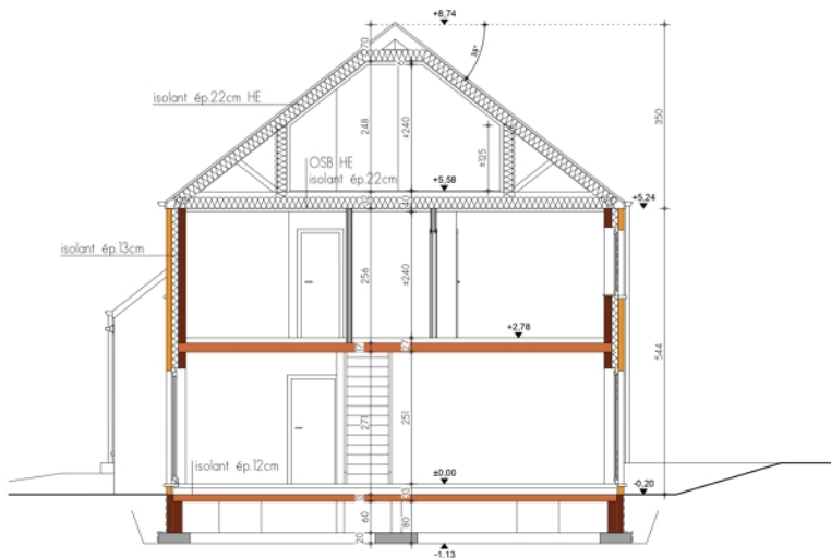
COUPE AA
