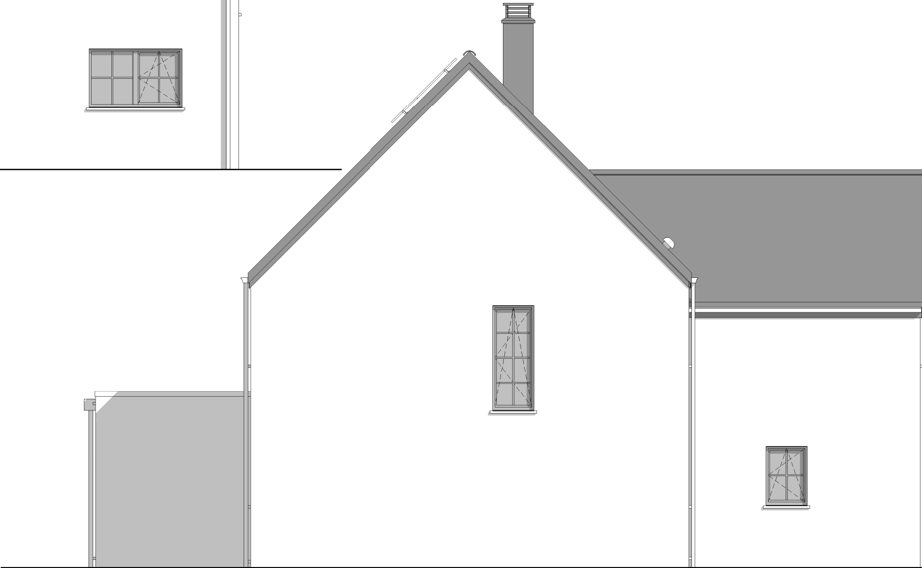
PIGNON GAUCHE
