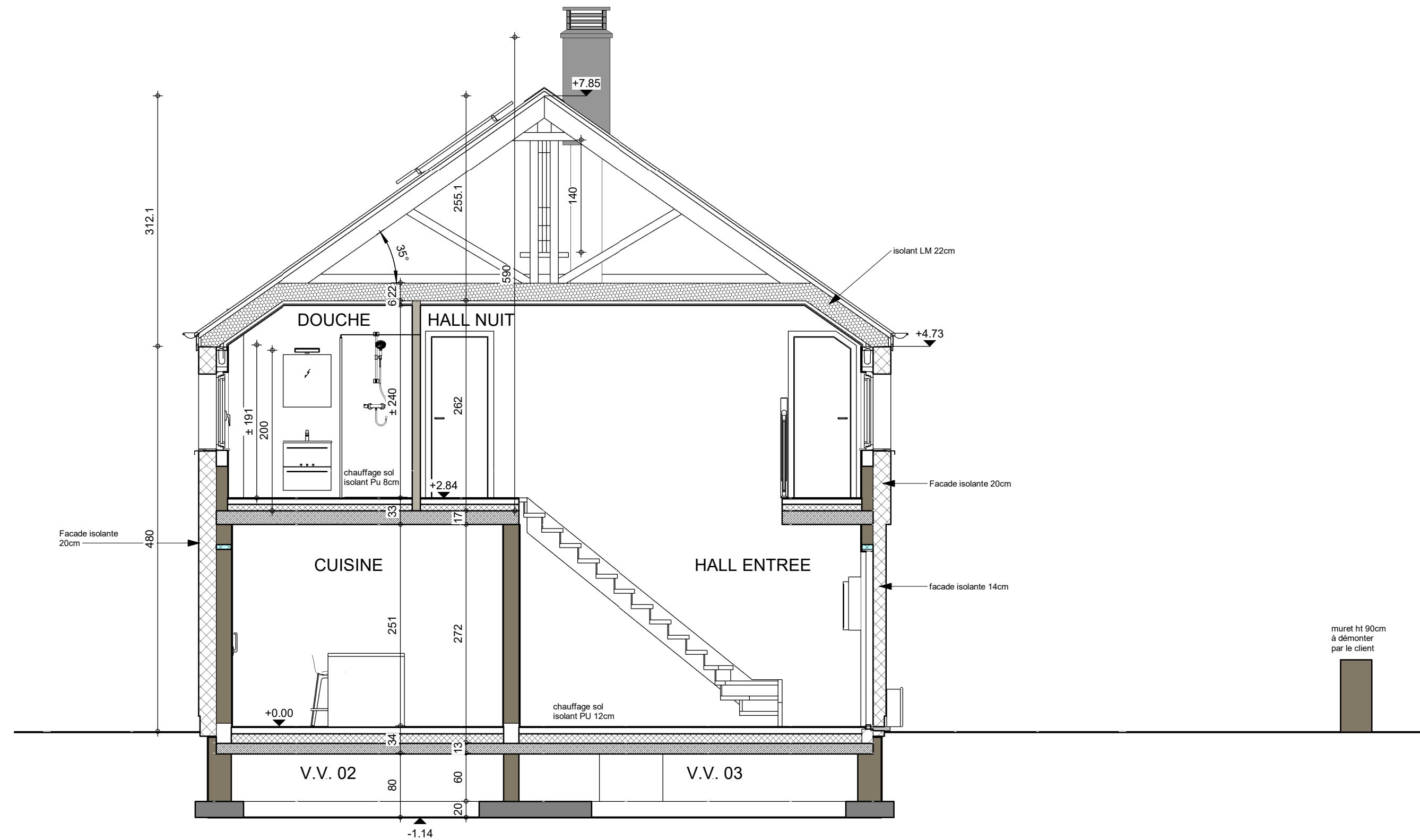
COUPE AA
