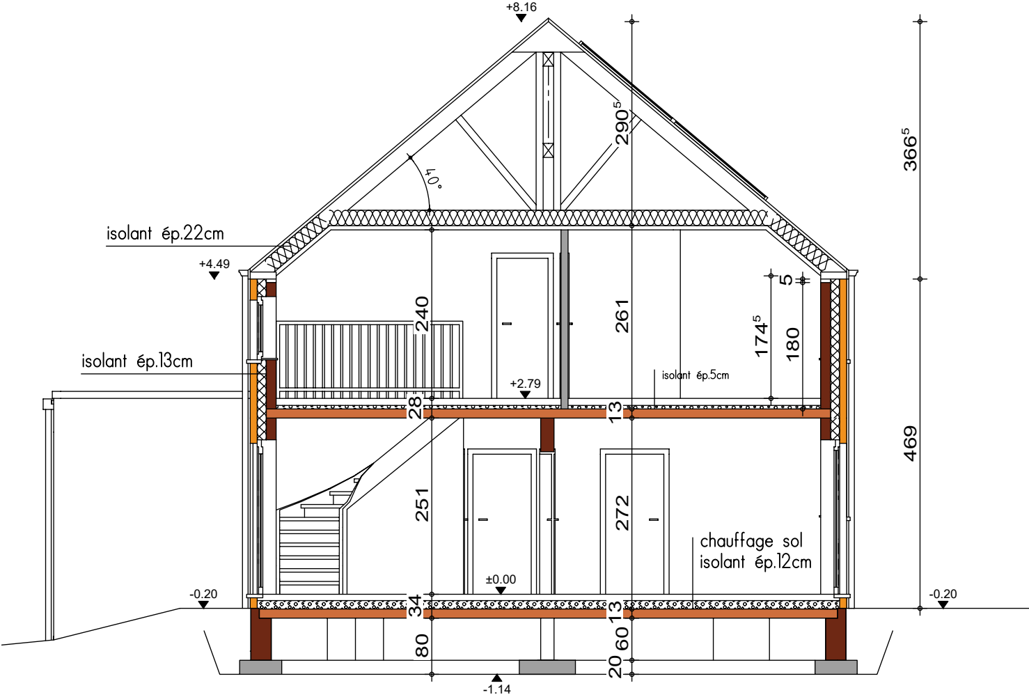
COUPE AA
