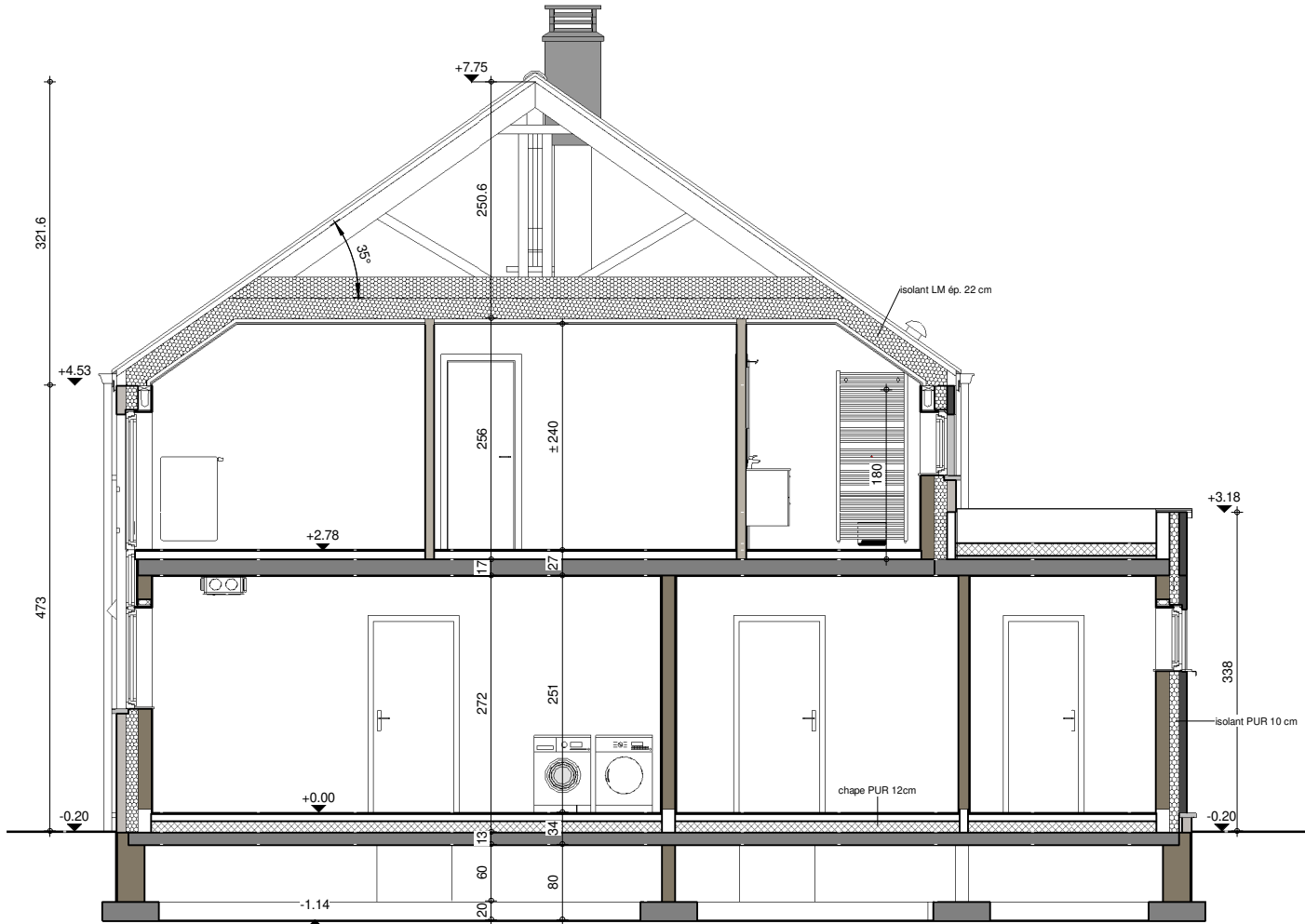
COUPE AA
