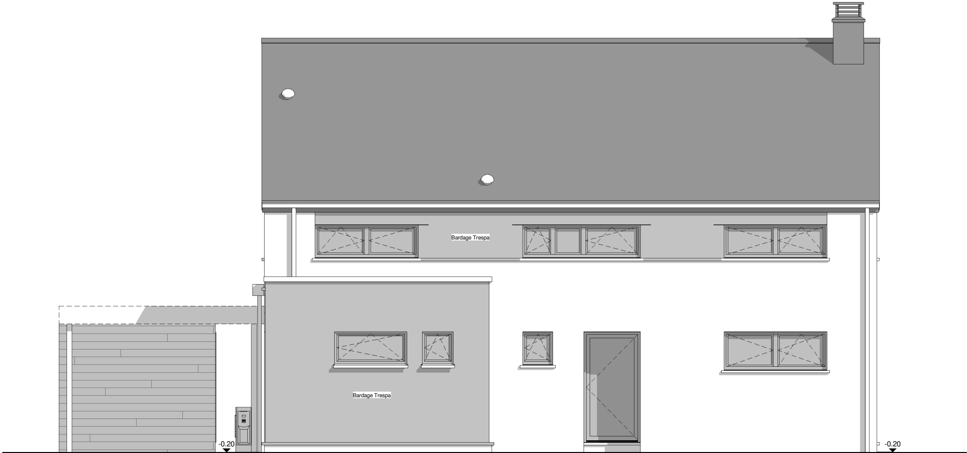
FACADE AVANT
