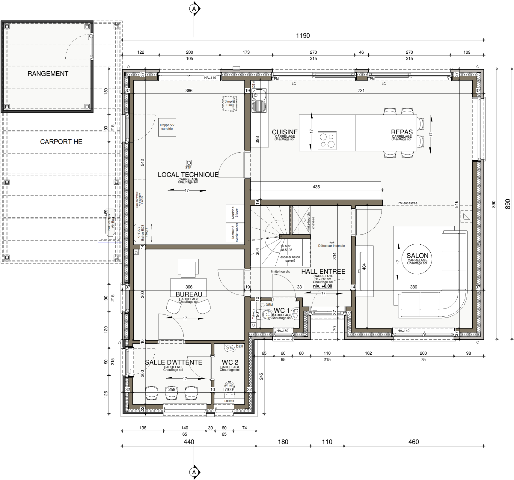
REZ-DE-CHAUSSEE
