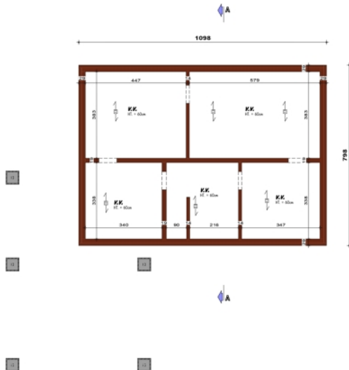
PLAN SOUS-SOL
