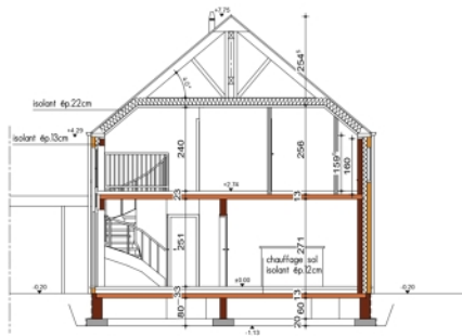
COUPE AA
