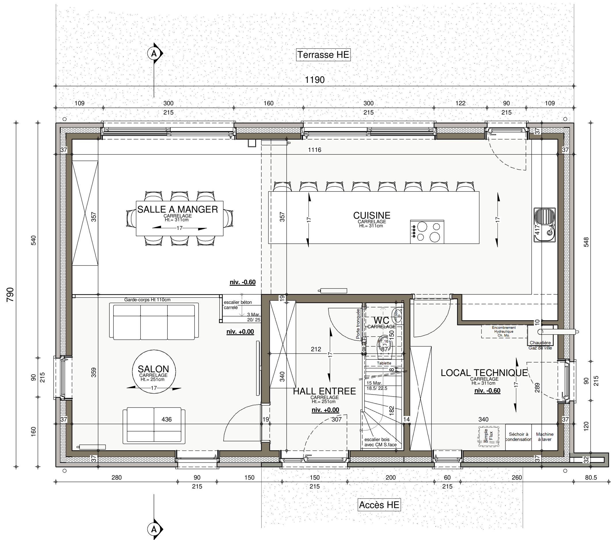
REZ-DE-CHAUSSEE
