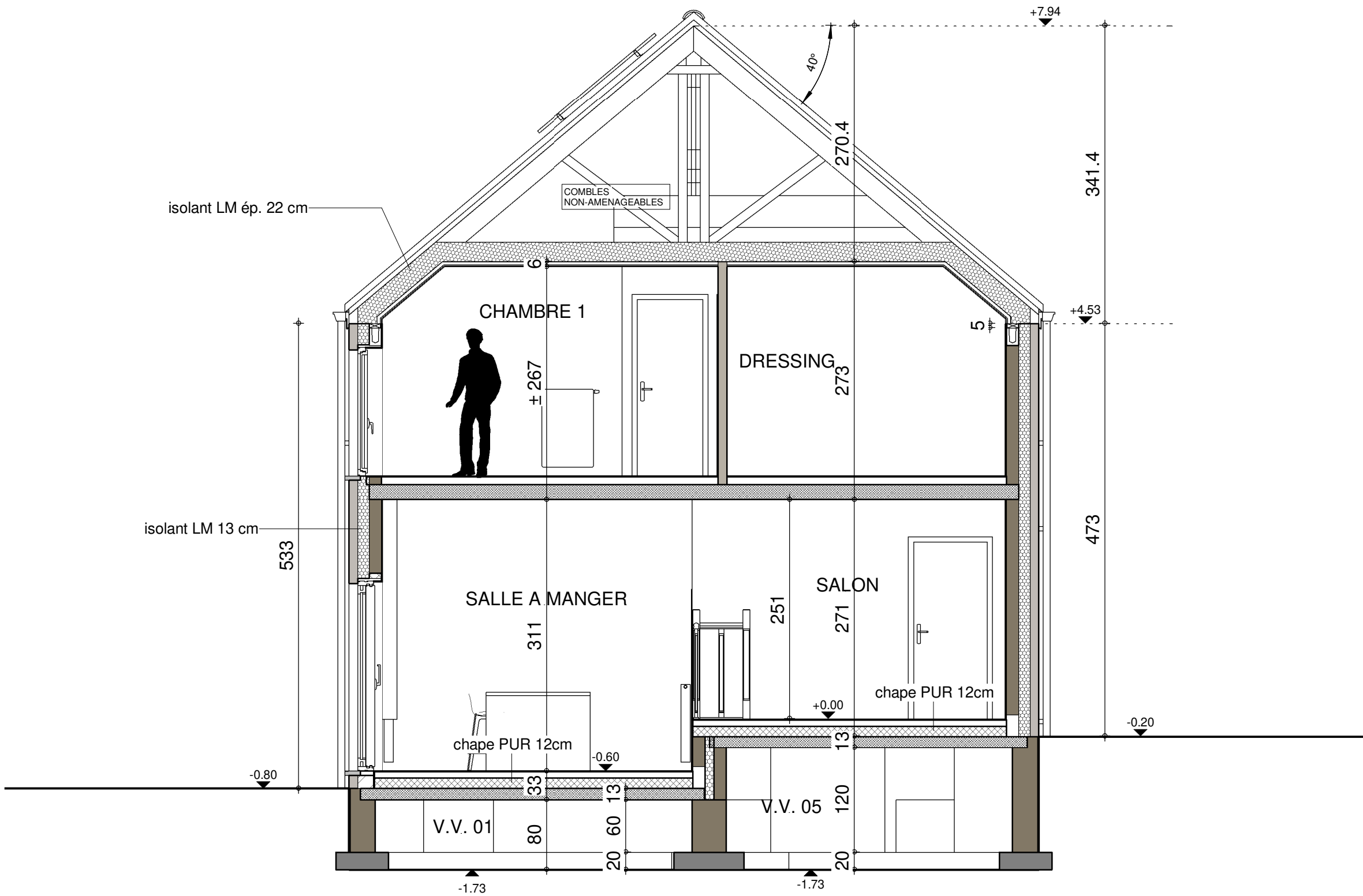
COUPE AA
