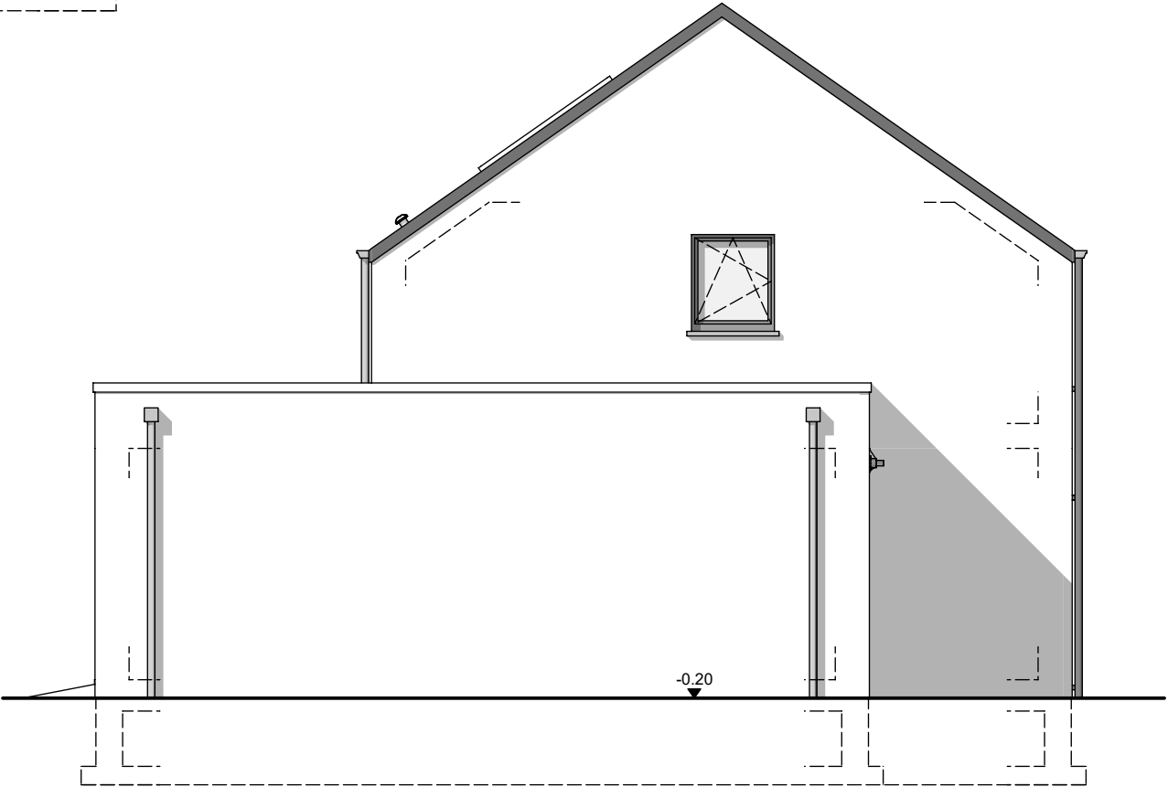
PIGNON DROIT
