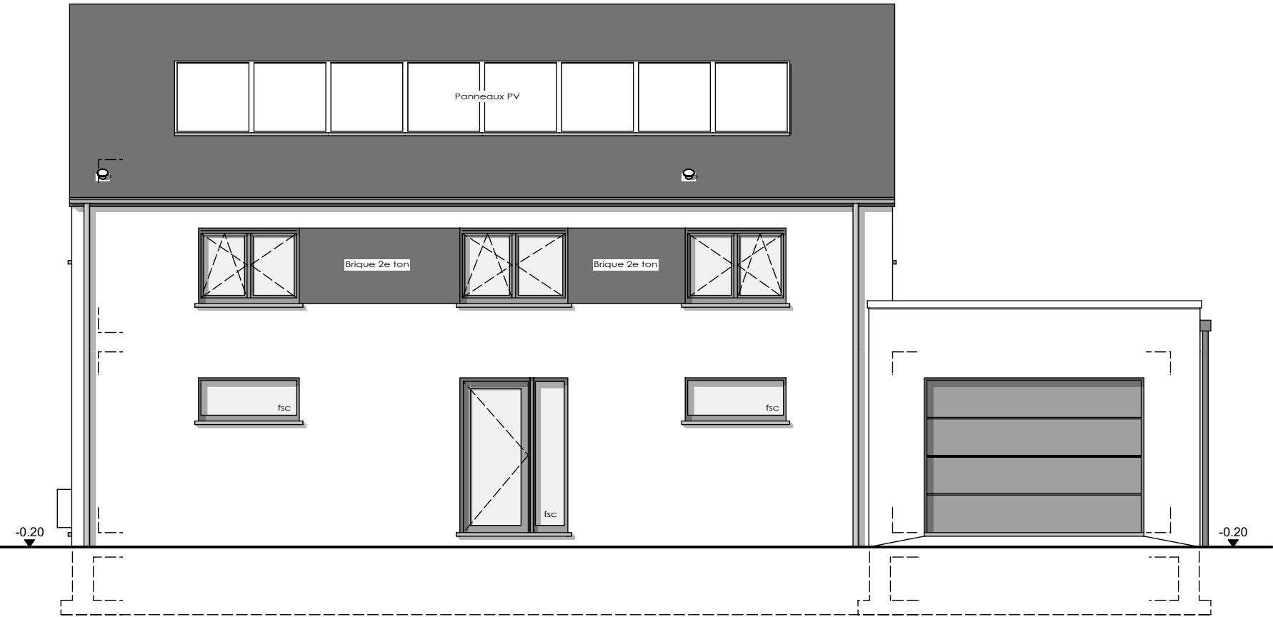
FACADE AVANT
