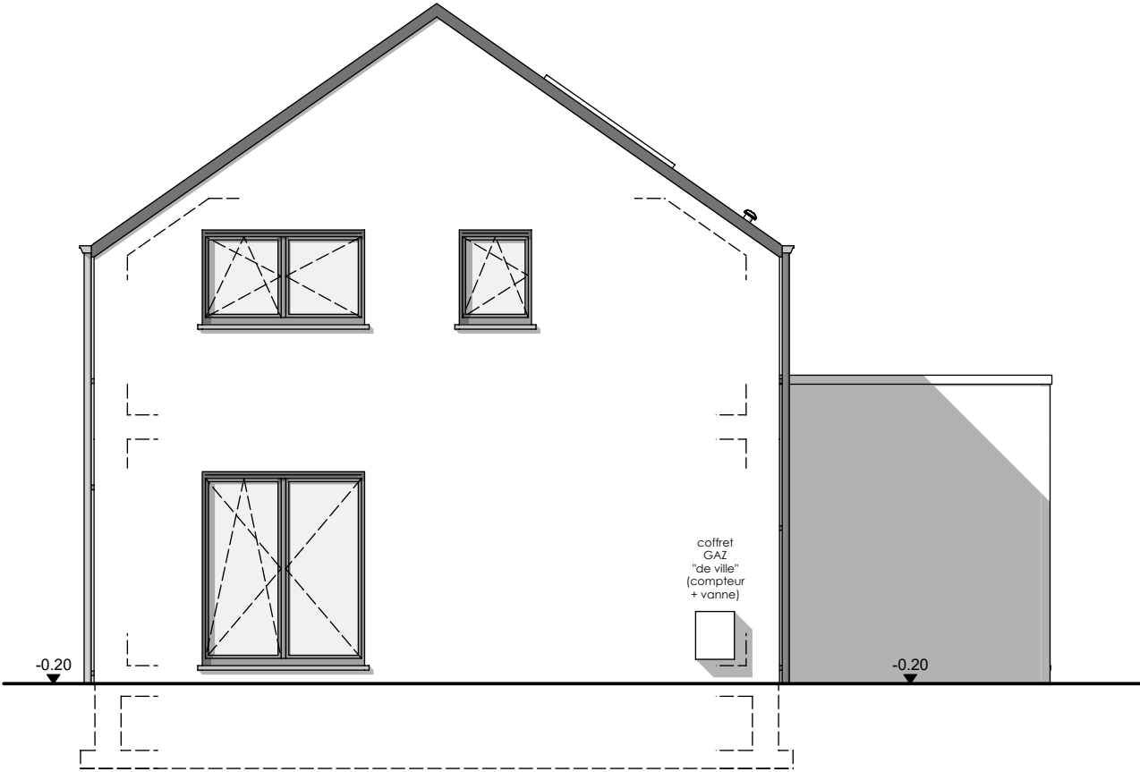
PIGNON GAUCHE
