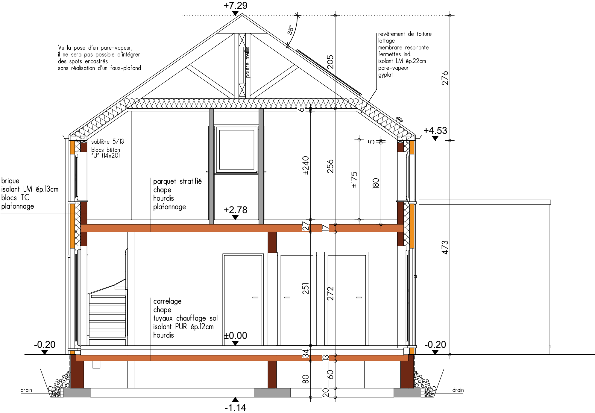
COUPE AA
