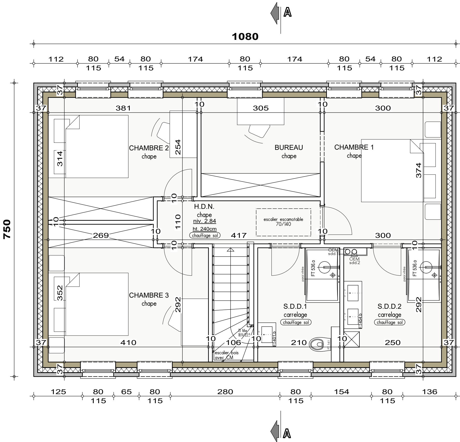
PLAN ETAGE
