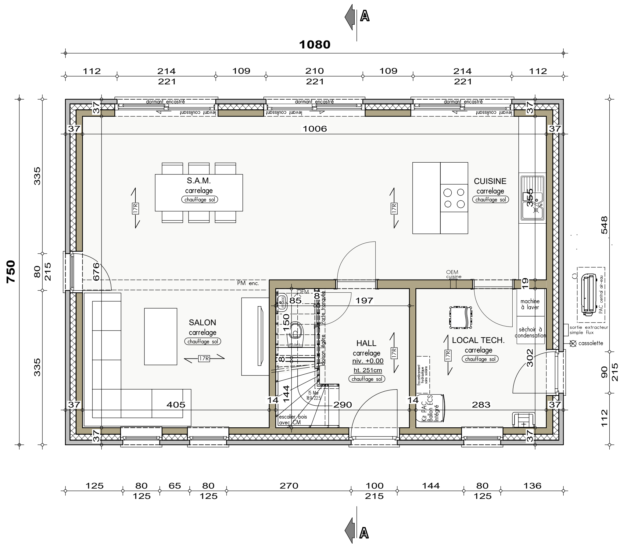
PLAN REZ-DE-CHAUSSEE
