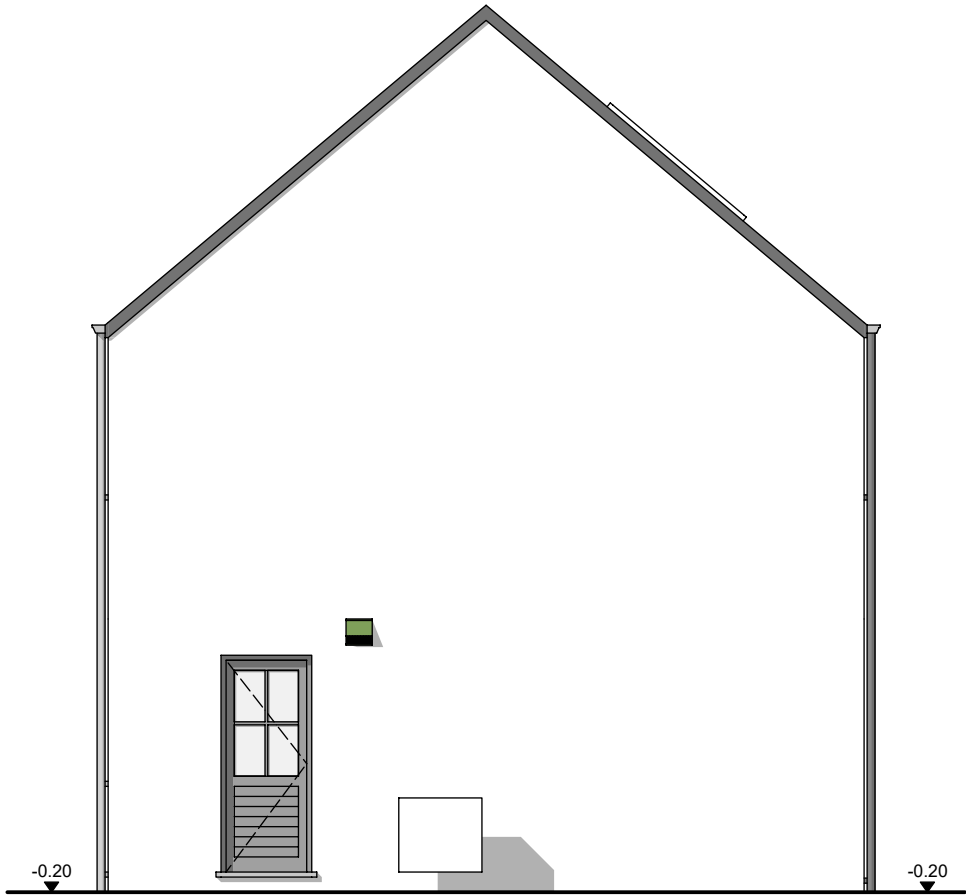
PIGNON DROIT
