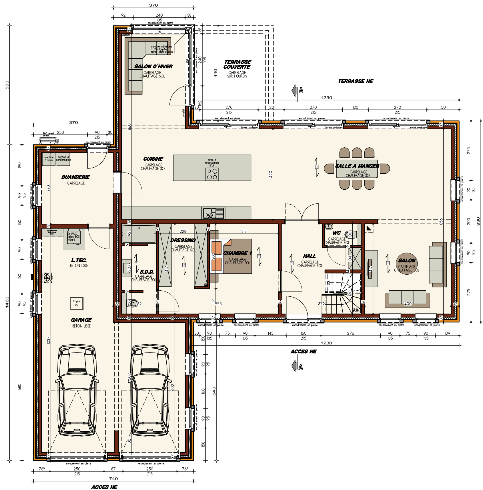
PLAN REZ-DE-CHAUSSEE
