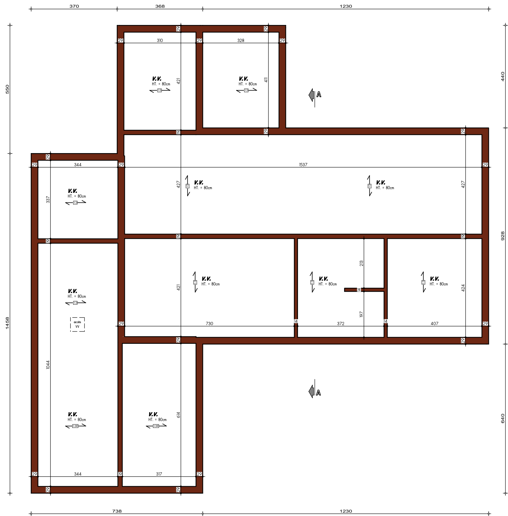
PLAN SOUS-SOL
