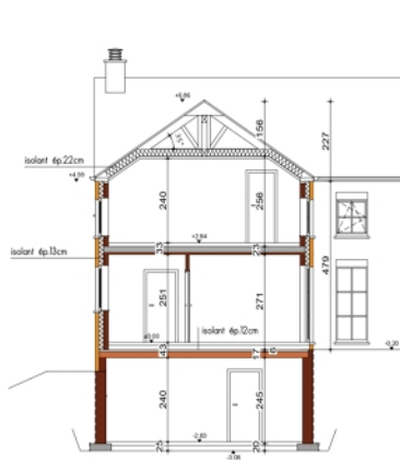
COUPE BB
