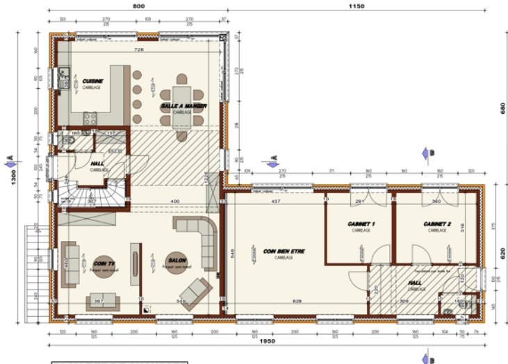
PLAN REZ-DE-CHAUSSÉE
