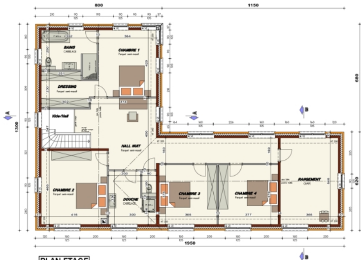
PLAN ETAGE
