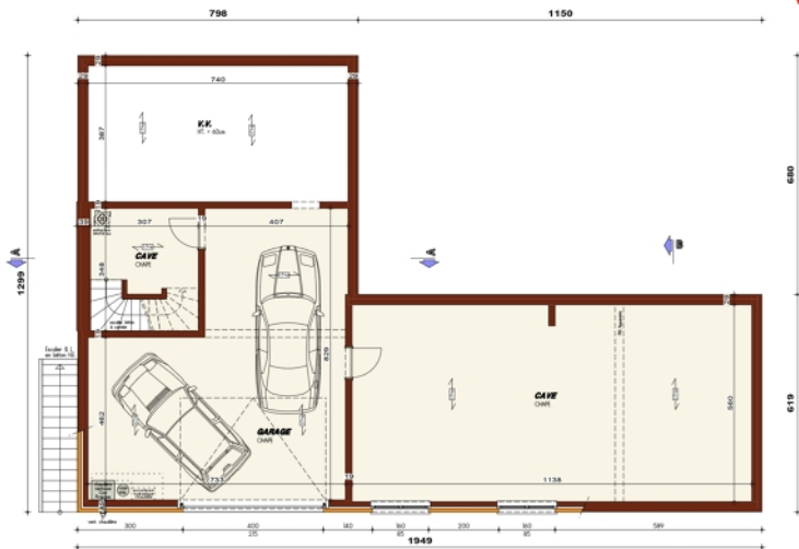
PLAN SOUS-SOL
