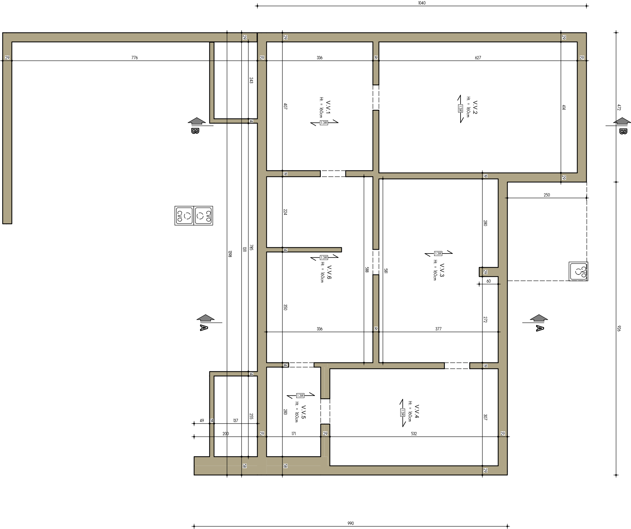
PLAN SOUS-SOL
