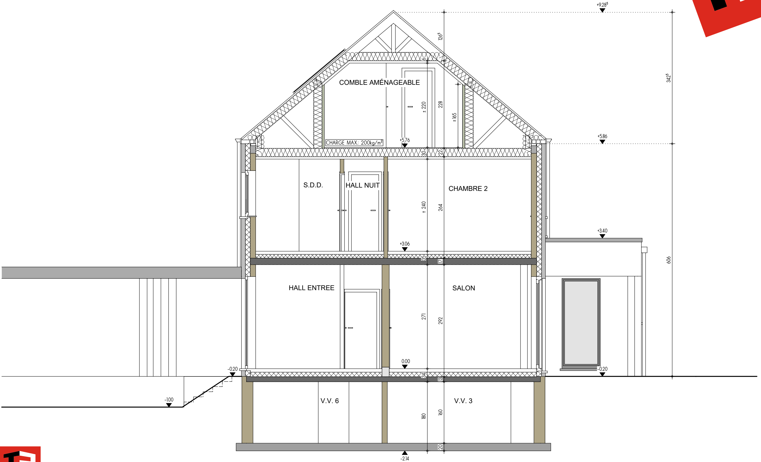
COUPE AA
