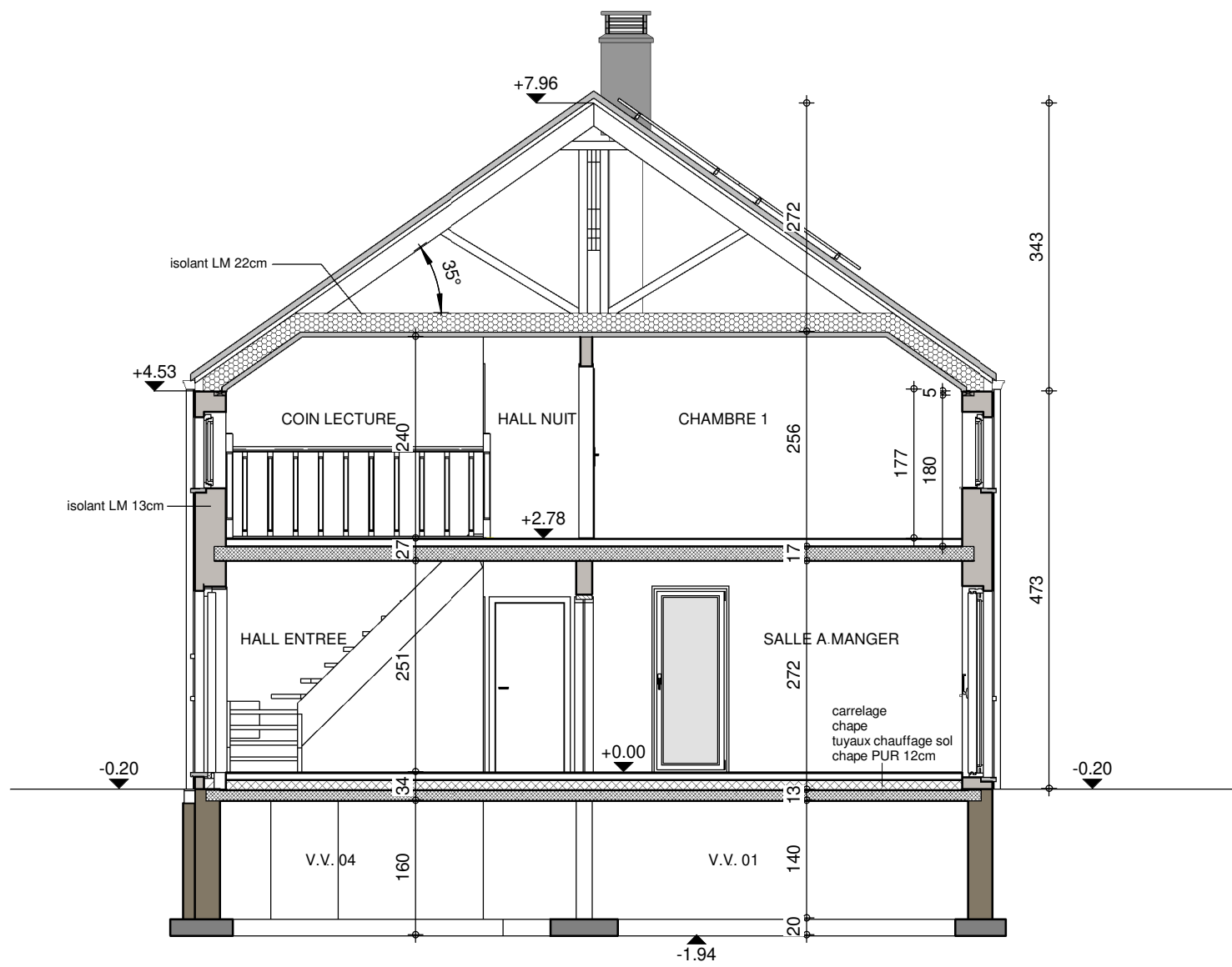
COUPE AA
