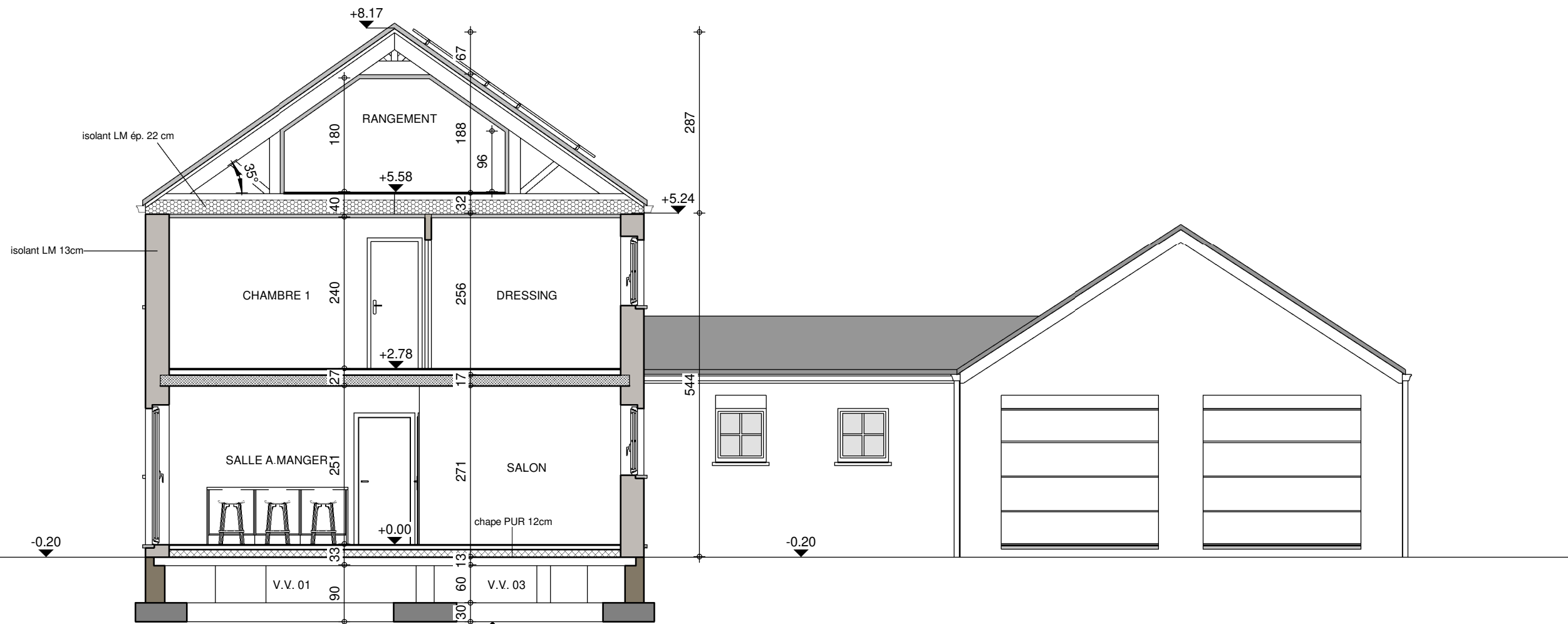
COUPE AA
