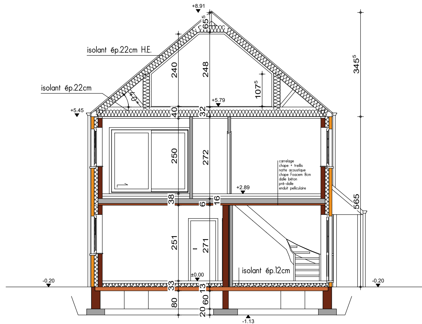
COUPE AA
