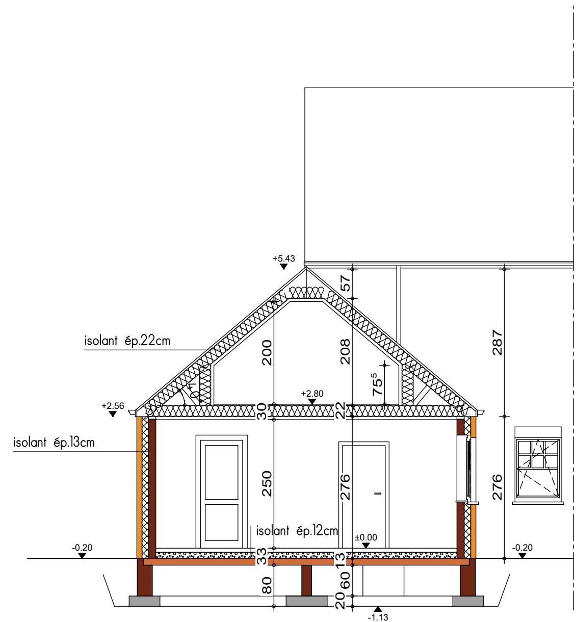
COUPE BB
