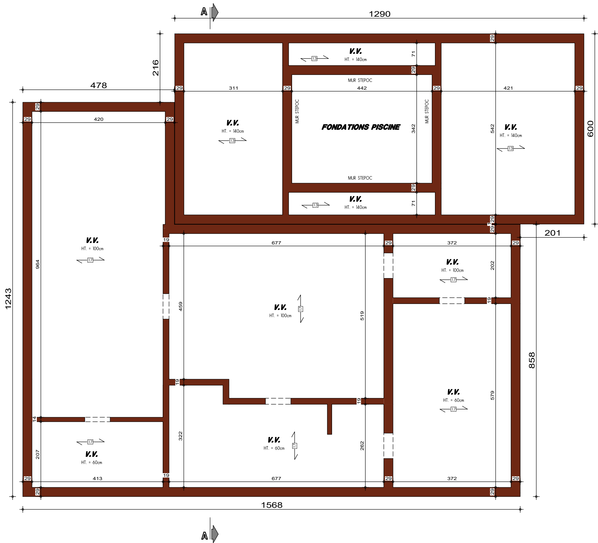
PLAN SOUS-SOL
