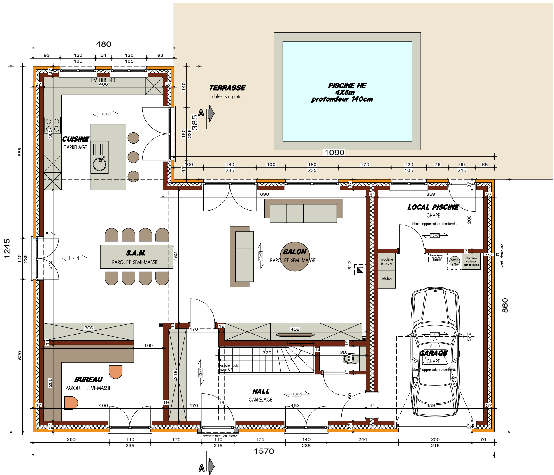
PLAN REZ-DE-CHAUSSEE
