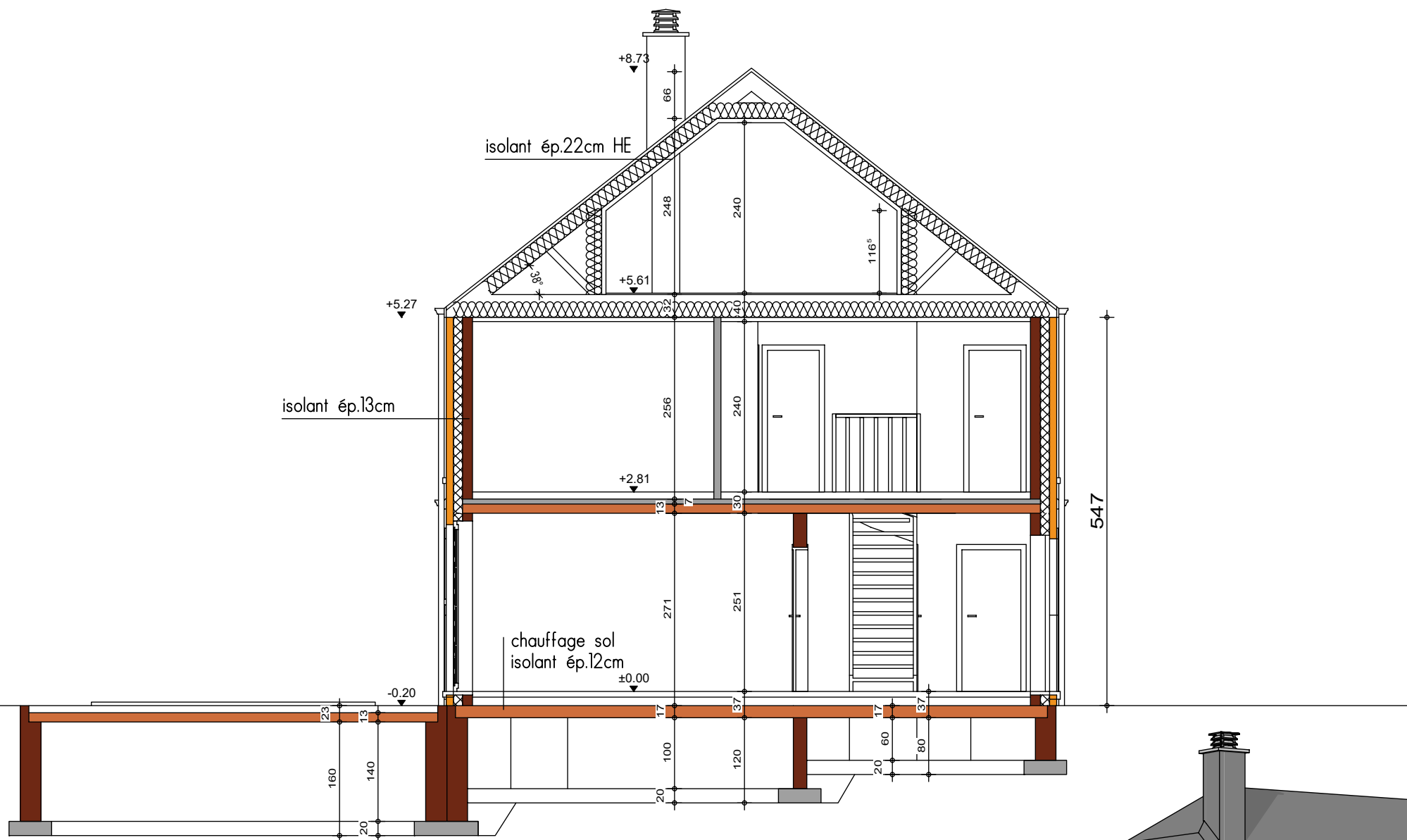
COUPE AA
